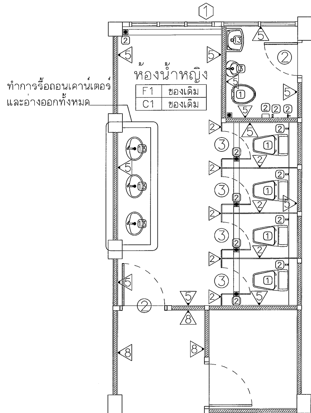
แปลนห้องน้ำหญิง ชั้นที่ 2 และ 3 เดิม Scale 1 : 50
