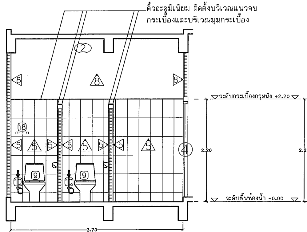
รูปตัดขยาย I Scale 1 : 50
