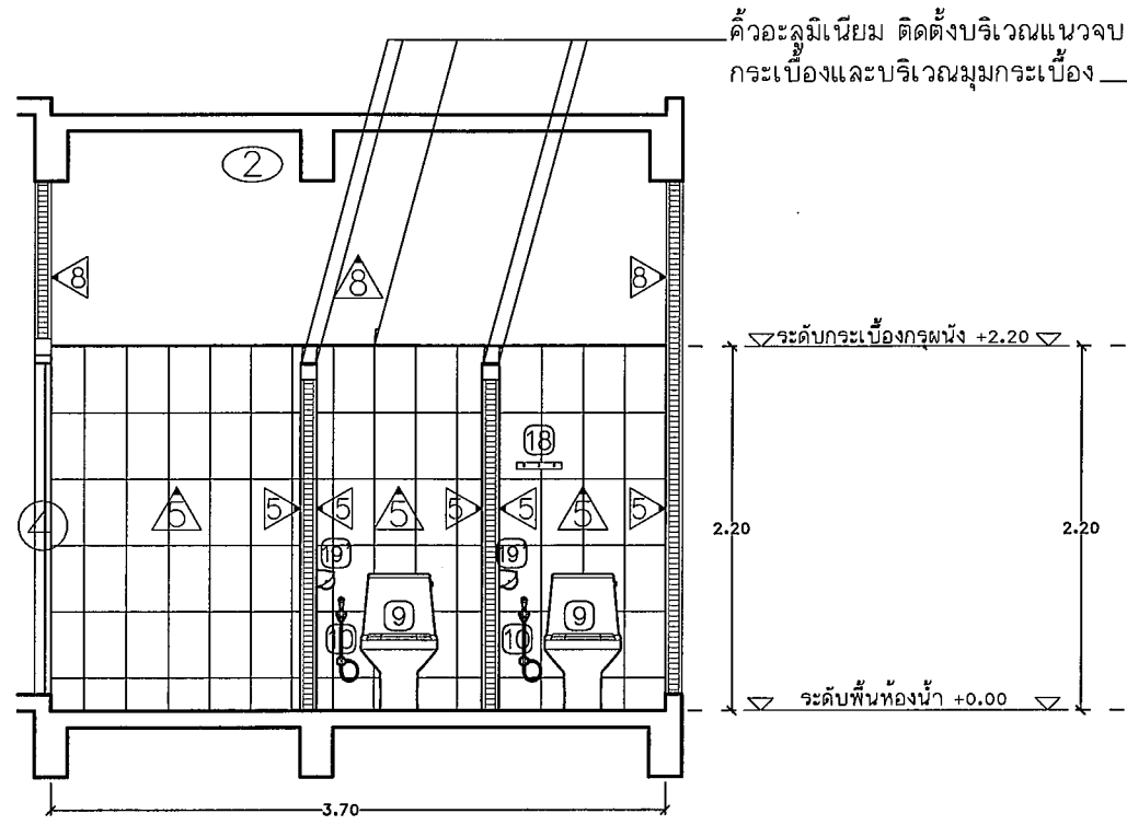
รูปตัดขยาย F Scale 1 : 50
