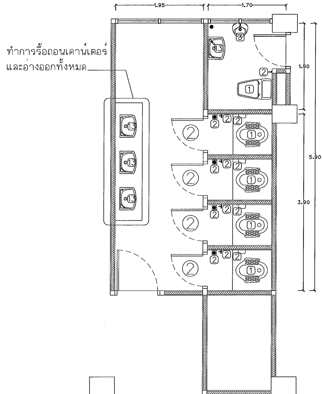
แปลนห้องน้ำหญิง ชั้นที่ 2 เดิม
