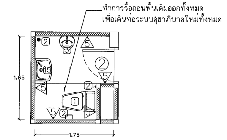
แปลนห้องน้ำอาจารย์ ชั้นที่ 1 ของเดิม Scale 1 : 50
