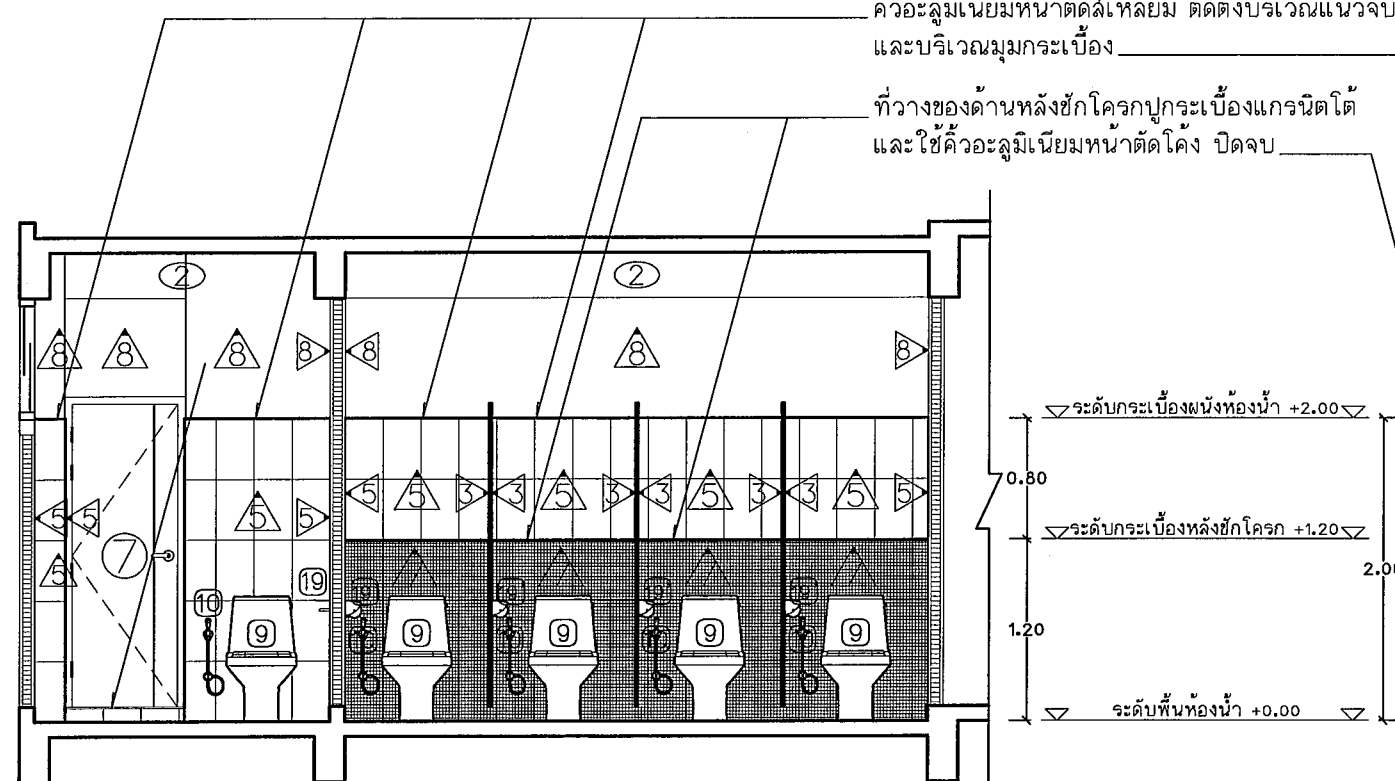
รูปตัดขยาย J Scale 1 : 50
