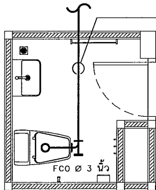
แปลนระบบน้ำโสโครกห้องน้ำอาจารย์ ชั้นที่ 1 Scale 1 : 50
