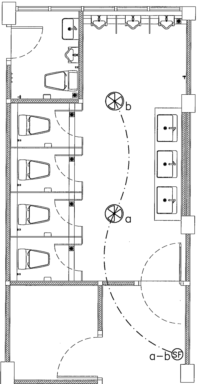
แปลนตำแหน่งพัฒมห้องน้ำชาย ชั้นที่ 2 Scale 1 : 50
