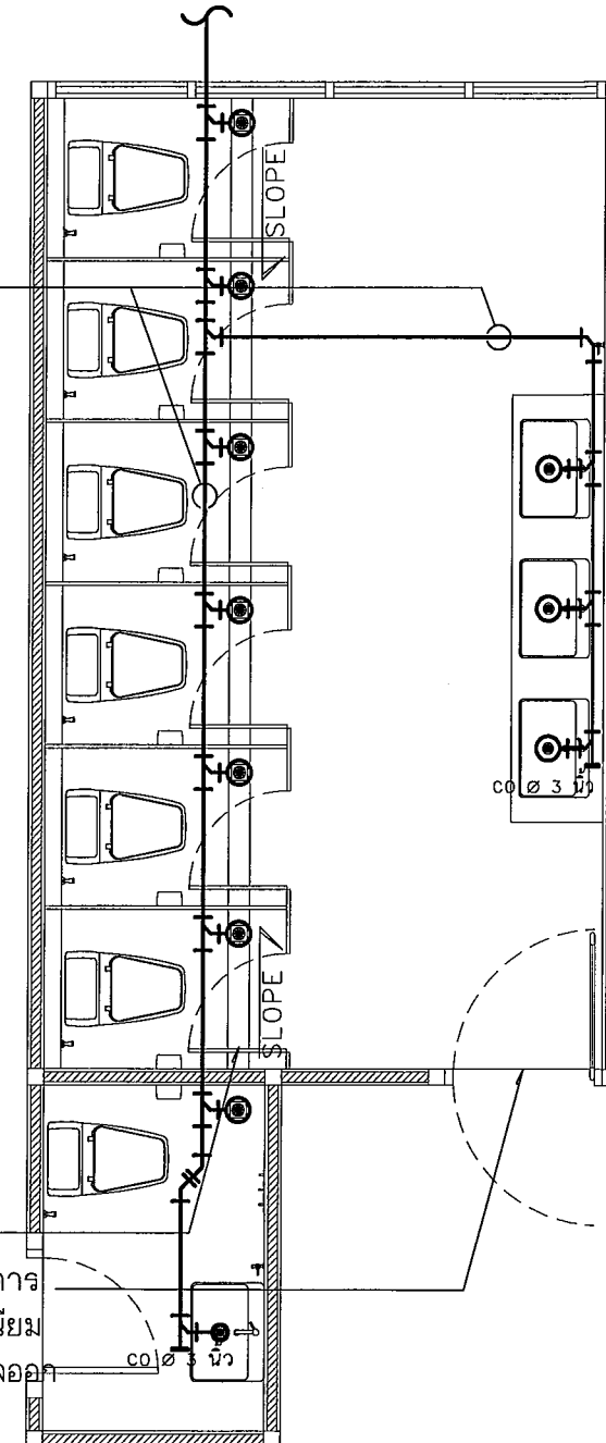
แปลนระบบน้ำทิ้งห้องน้ำหญิง ชั้นที่ 2 และ 3 Scale 1 : 50
