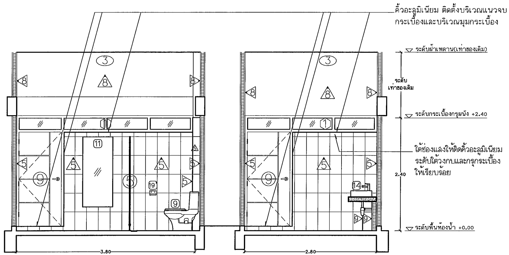
รูปตัดขยาย B Scale 1 : 50
