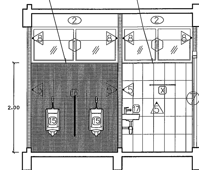
รูปตัดขยาย I Scale 1 : 50
