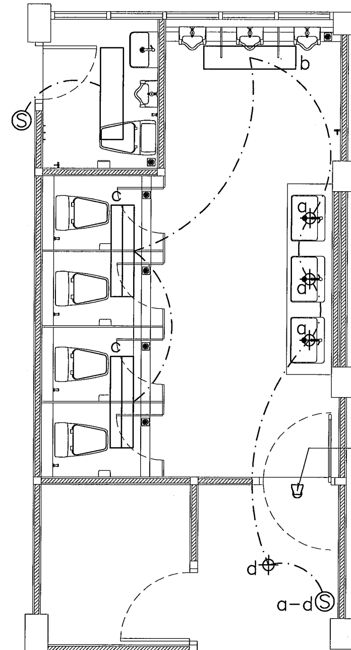
แปลนระบบไฟฟ้าแสงสว่างห้องน้ำชาย ชั้นที่ 2 Scale 1 : 50
