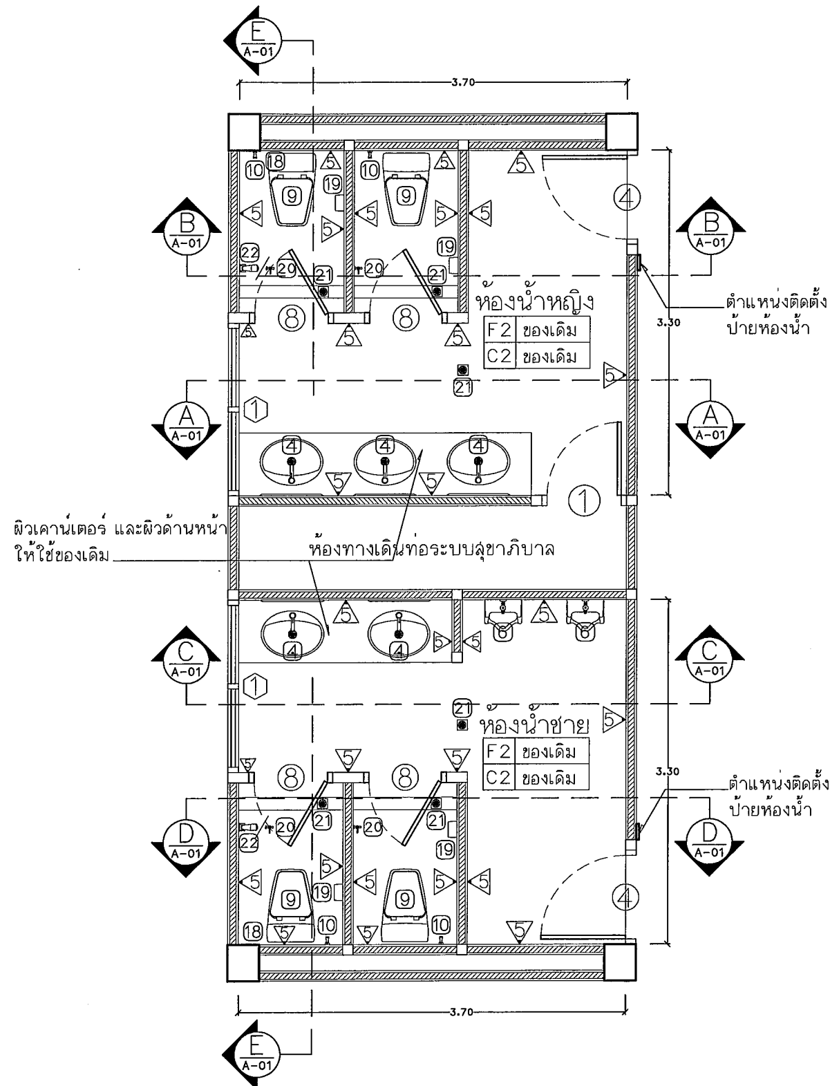
แปลนห้องน้ำชาย-หญิงชั้น 1, 2 และ 3 (ทิศเหนือ) แบบปรับปรุง Scale 1 : 50
