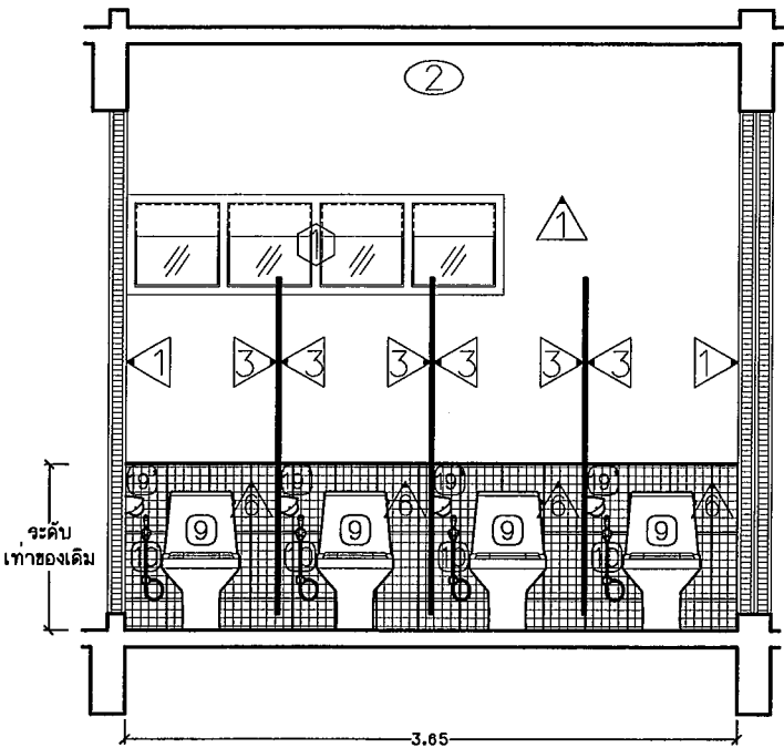
รูปตัดขยาย C Scale 1 : 50
