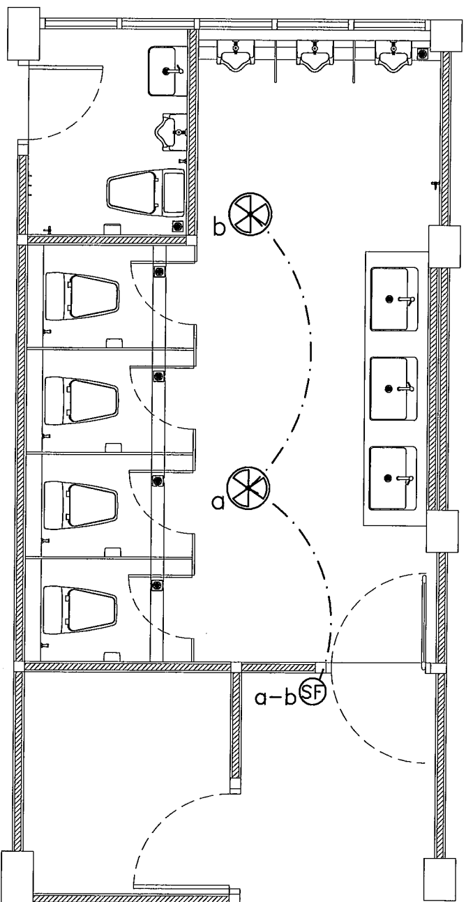
แปลนตำแหน่งพัฒมห้องน้ำชาย ชั้นที่ 2 และ 3 Scale 1 : 50
