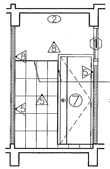
รูปตัด E Scale 1 : 50
