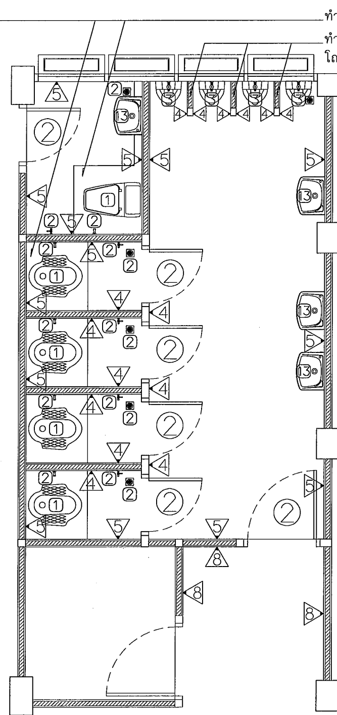
แปลนห้องน้ำชาย ชั้นที่ 2 และ 3 เดิม Scale 1 : 50
