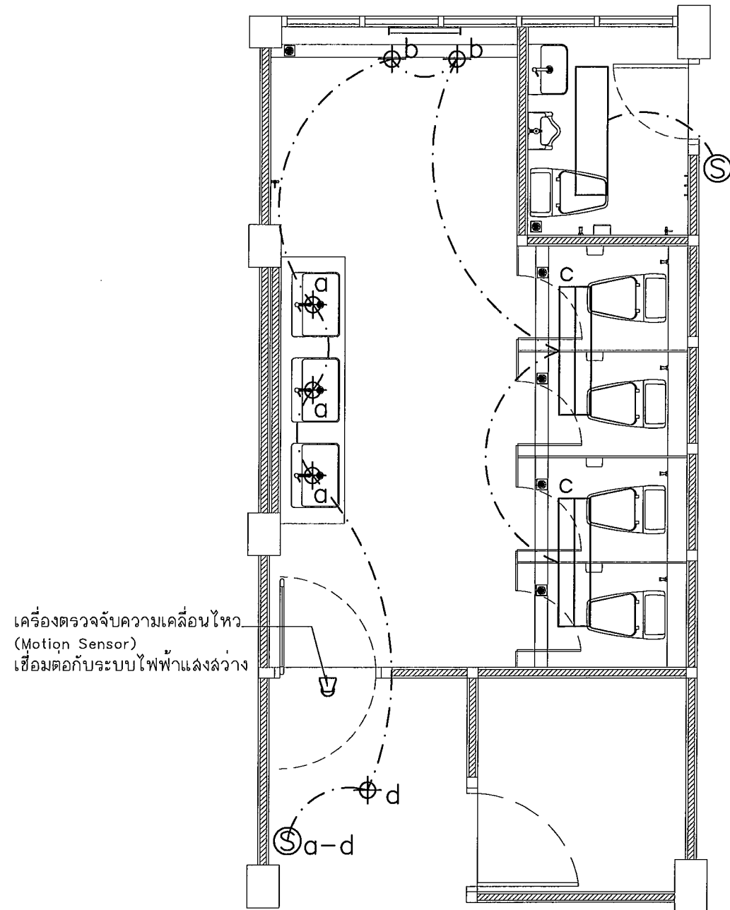
แปลนระบบไฟฟ้าแสงสว่างห้องน้ำหญิง ชั้นที่ 2 และ 3 Scale 1 : 50
