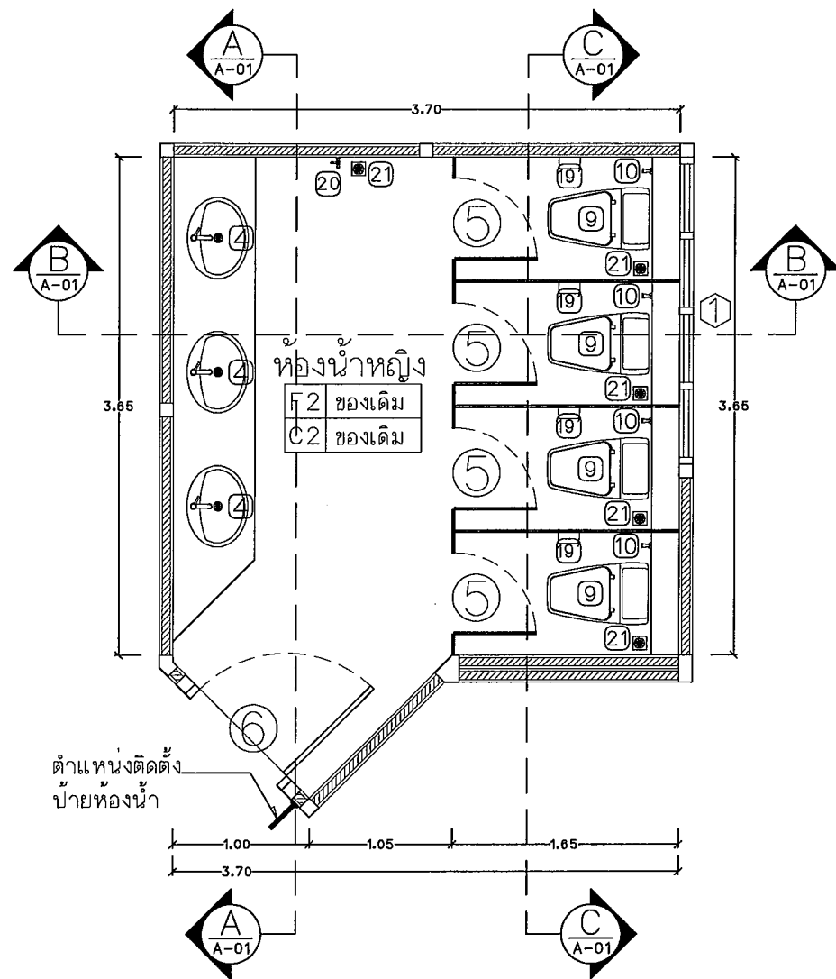
แปลนห้องน้ำห้องน้ำชั้นที่ 1-9 แบบปรับปรุง Scale 1 : 50
