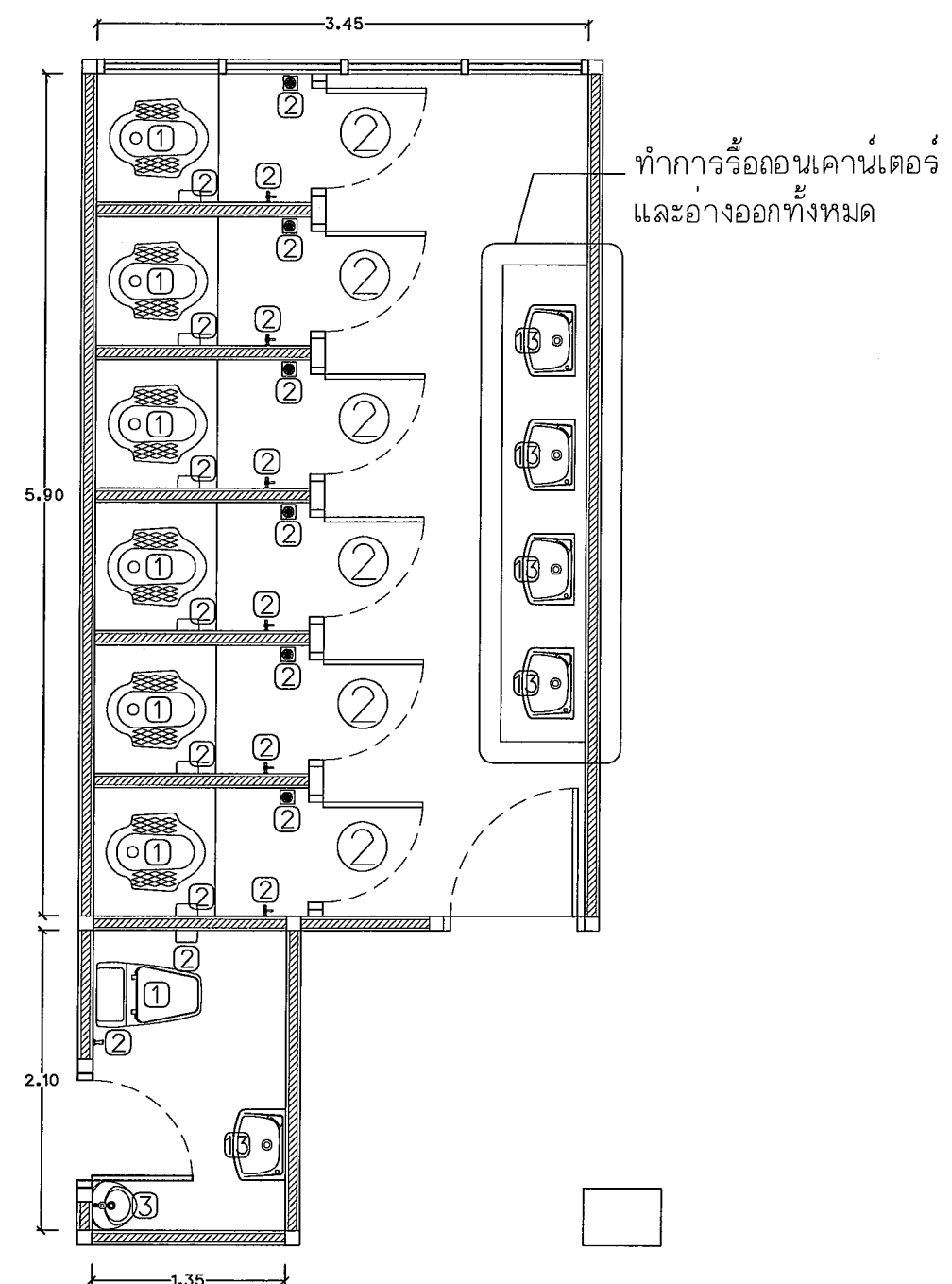
แปลนห้องน้ำหญิง ชั้นที่ 2 และ 3 เดิม
