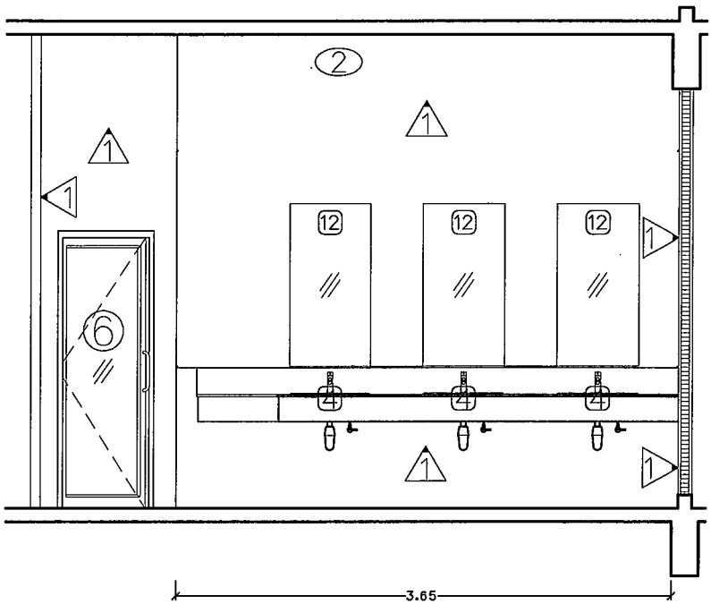
รูปตัดขยาย A Scale 1 : 50
