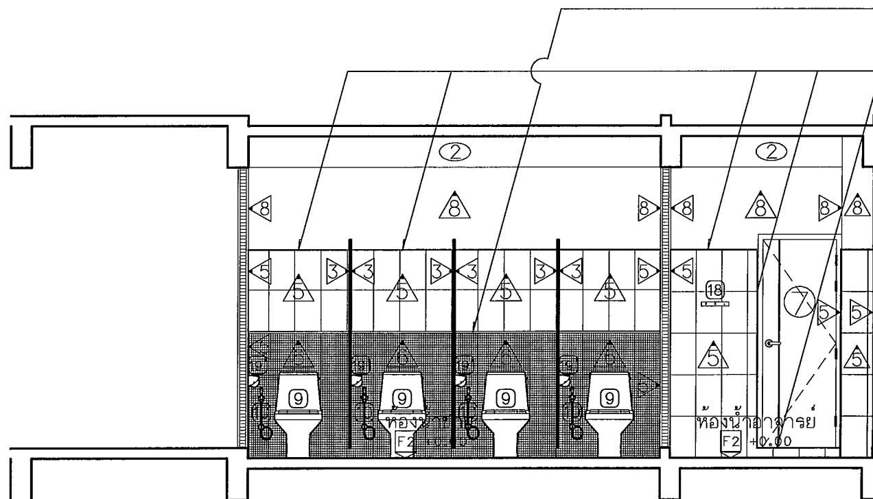
รูปตัดขยาย G Scale 1 : 50
