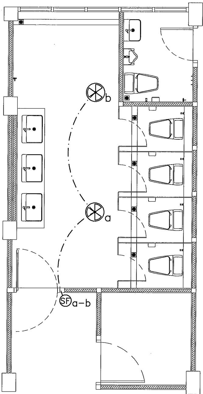
แปลนตำแหน่งพัฒมห้องน้ำหญิง ชั้นที่ 2 และ 3 Scale 1 : 50
