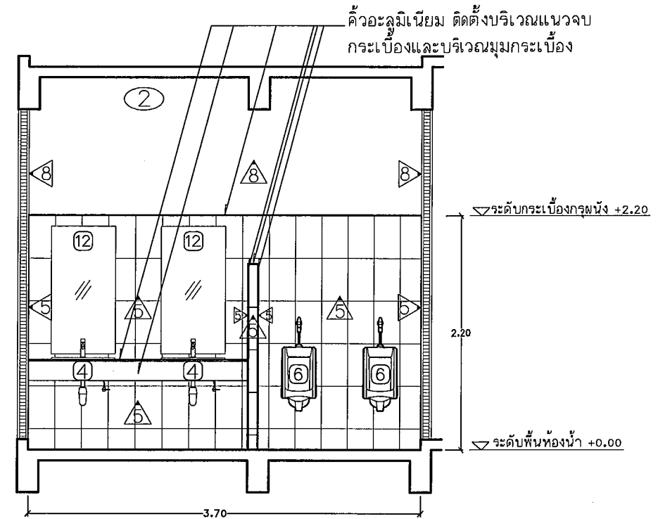
รูปตัดขยาย C Scale 1 : 50
