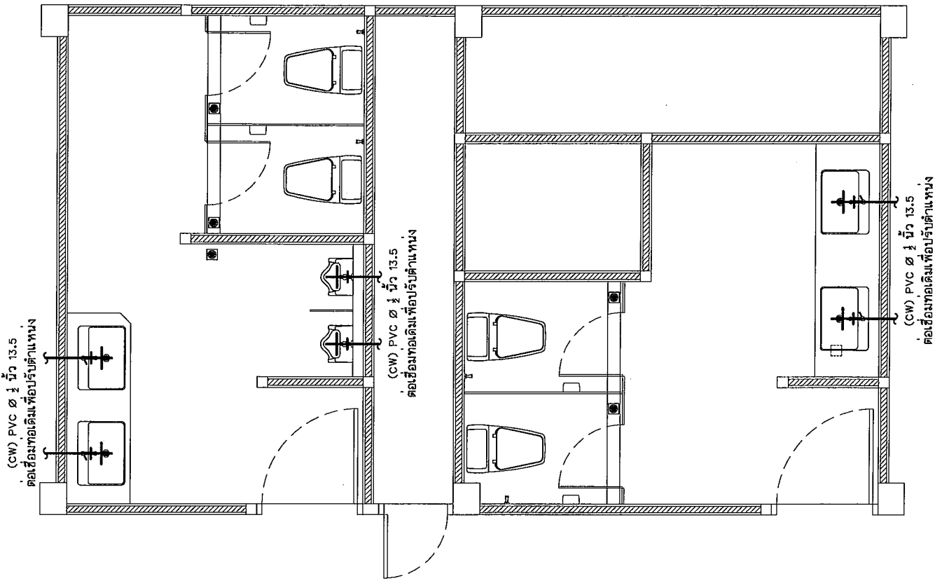
แปลนระบบน้ำดี ห้องน้ำห้องประชุมควาลัย Scale 1 : 50
