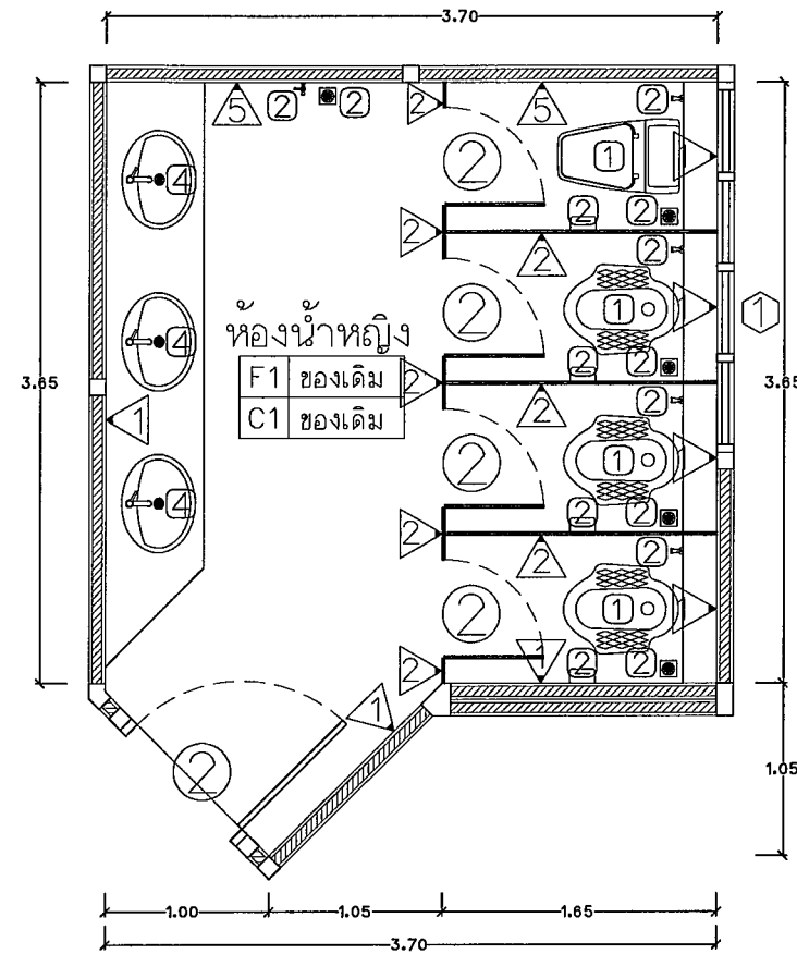
แปลนห้องน้ำหญิง ชั้นที่ 1-9 เดิม Scale 1 : 50
