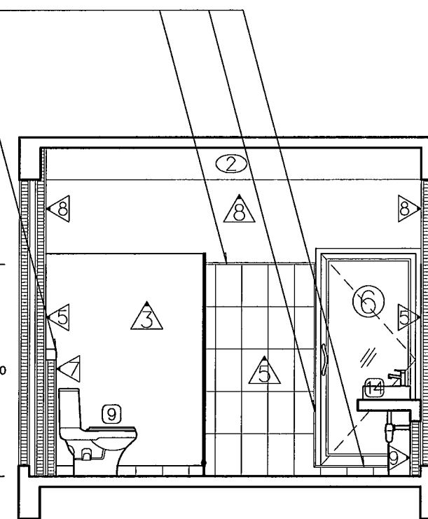
รูปตัดขยาย K Scale 1 : 50
