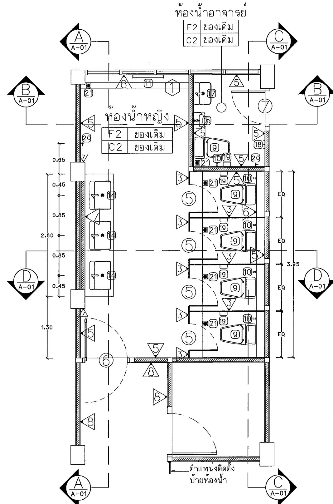
แปลนห้องน้ำหญิงชั้นที่ 2 และ 3 แบบปรับปรุง
