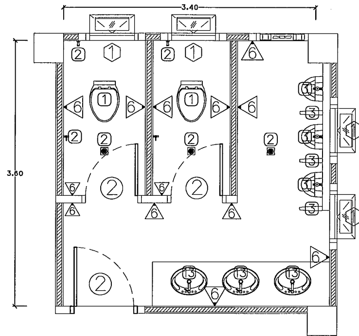
แปลนห้องน้ำชายโรงเรียนลำอิตา ชั้นที่ 1-3 แบบเดิม Scale 1 : 50
