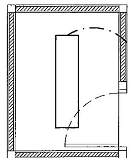
แปลนระบบไฟฟ้าแสงสว่างห้องเก็บของ ชั้นที่ 1 Scale 1 : 50
