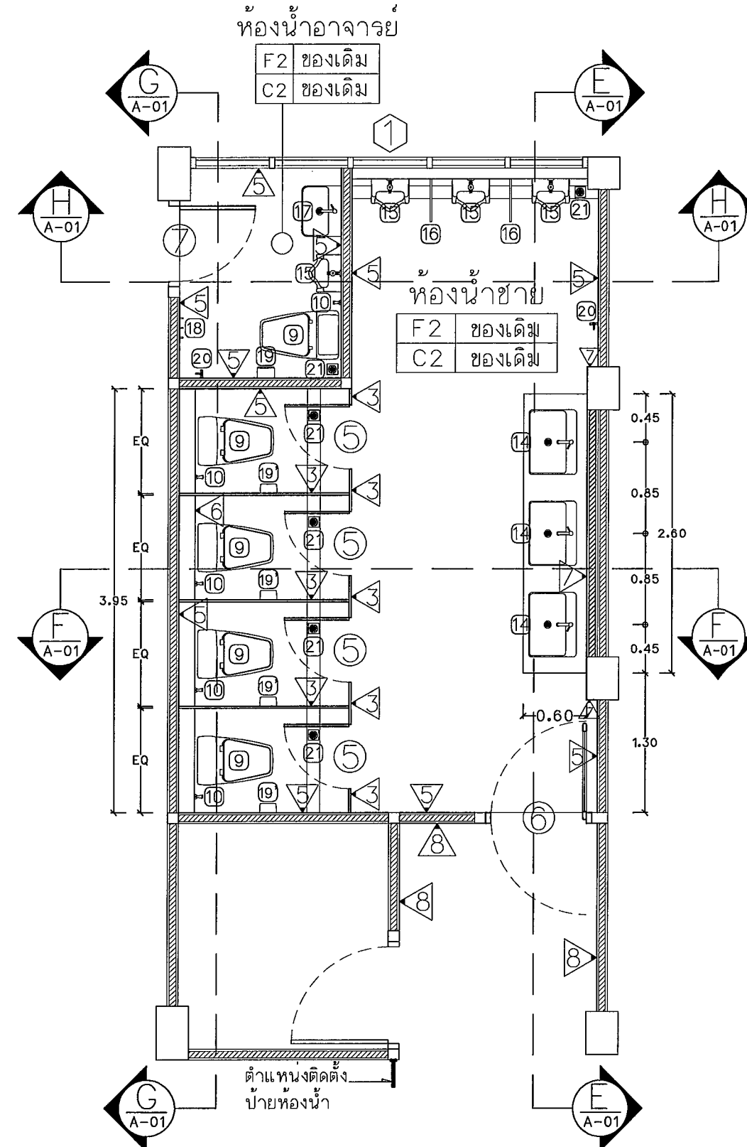
แปลนห้องน้ำชายชั้นที่ 2 แบบปรับปรุง
