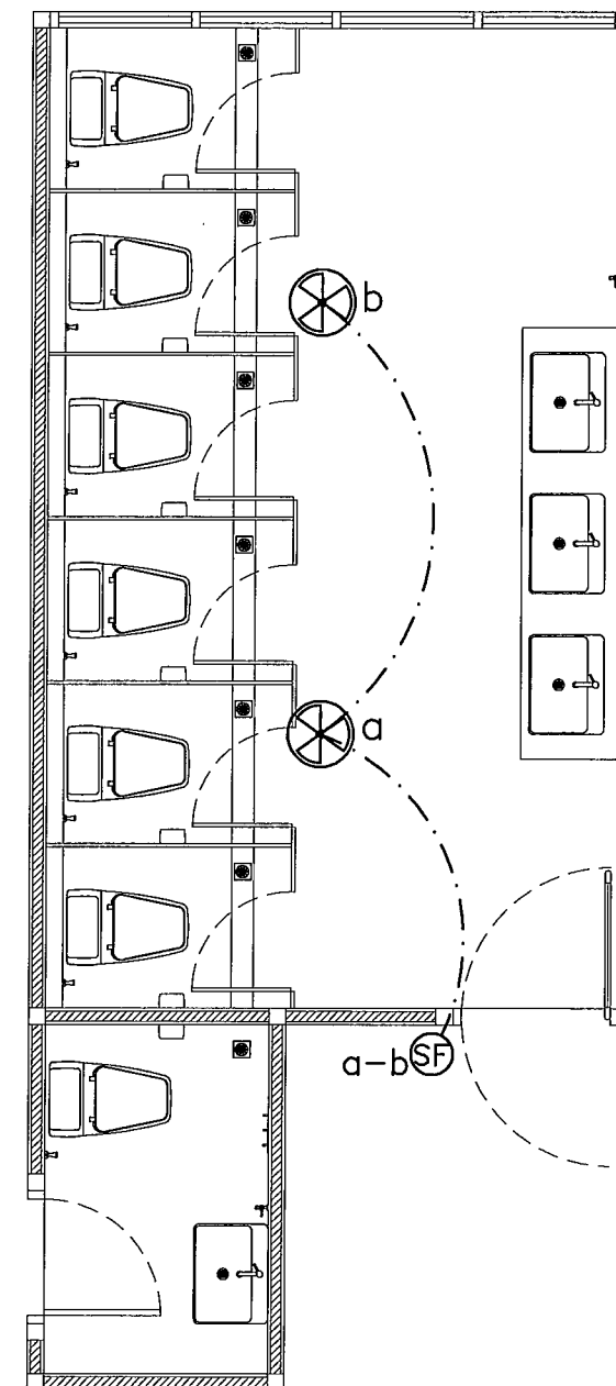
แปลนตำแหน่งพัฒมห้องน้ำหญิง ชั้นที่ 2 และ 3 Scale 1 : 50
