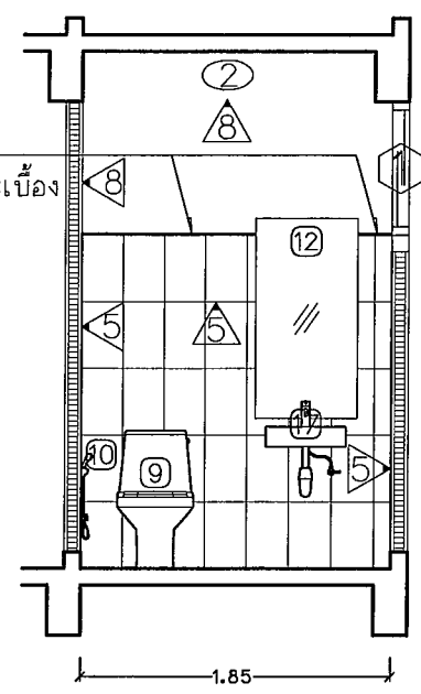
รูปตัด A Scale 1 : 50
