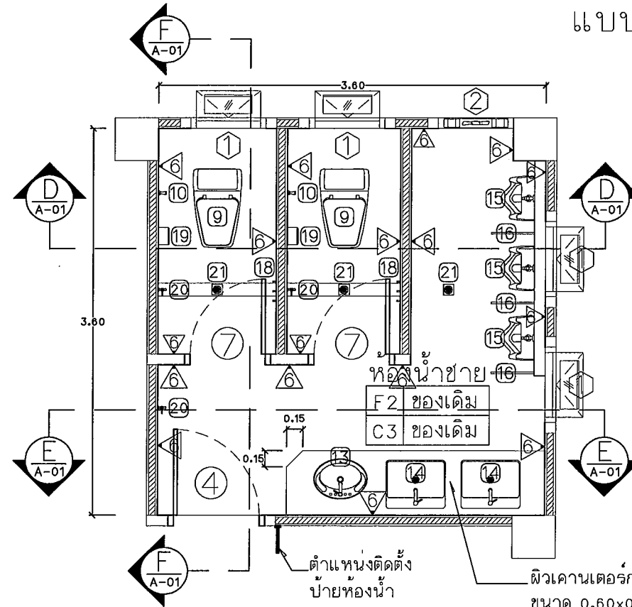
แปลนห้องน้ำชายโรงเรียนลำอิตา ชั้นที่ 1-2 แบบปรับปรุง Scale 1 : 50
