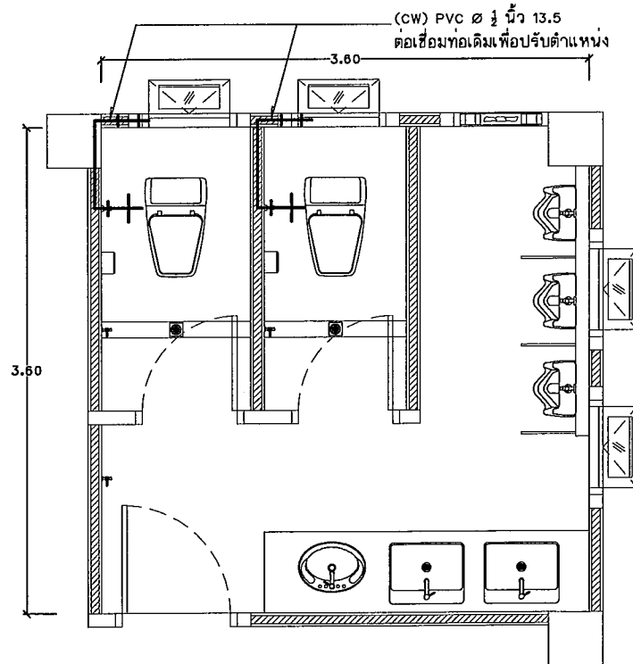
แปลนระบบน้ำดีห้องน้ำชายโรงเรียนลำอีต๊ะ ชั้นที่ 1-3 Scale 1 : 50
