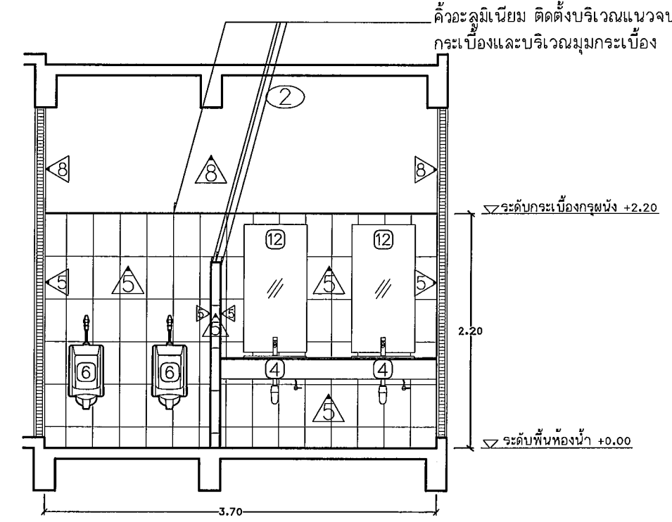
รูปตัดขยาย H Scale 1 : 50
