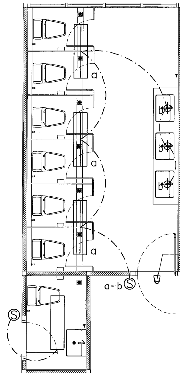
แปลนระบบไฟฟ้าแสงสว่างห้องน้ำหญิง ชั้นที่ 2 และ 3 Scale 1 : 50
