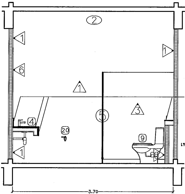
รูปตัดขยาย B Scale 1 : 50
