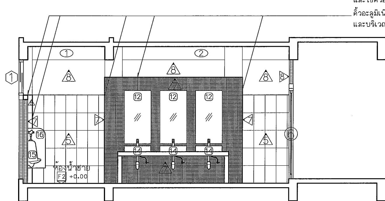
รูปตัดขยาย E Scale 1 : 50
