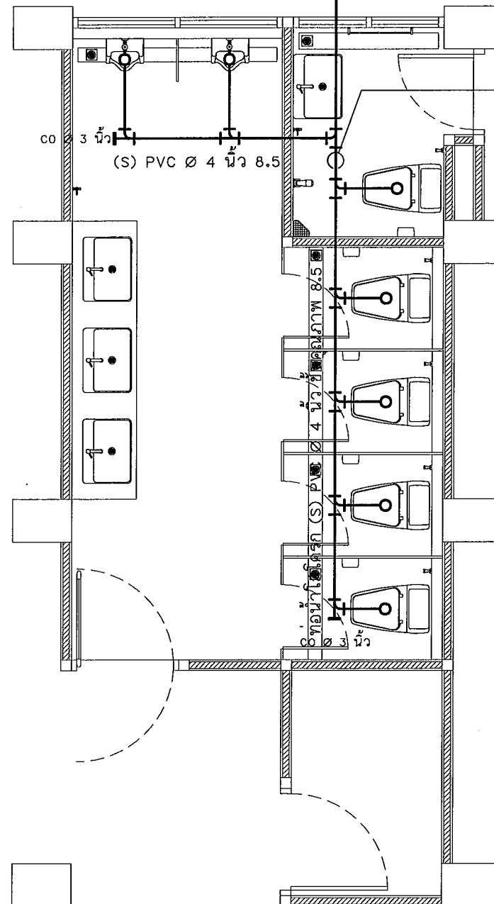
แปลนระบบน้ำโสโครกห้องน้ำชาย ชั้นที่ 2 Scale 1 : 50
