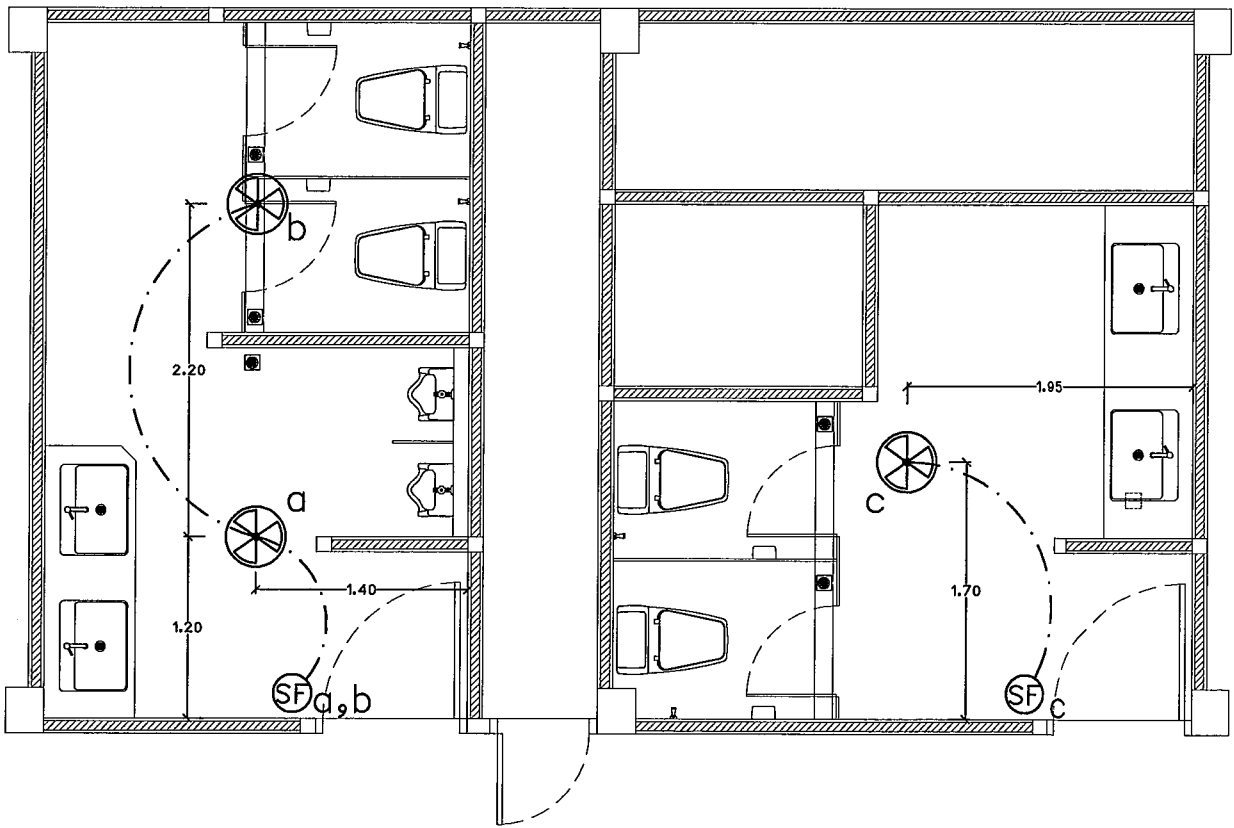
แปลนตำแหน่งพัดลม ห้องน้ำห้องประชุมควิลัย Scale 1 : 50
