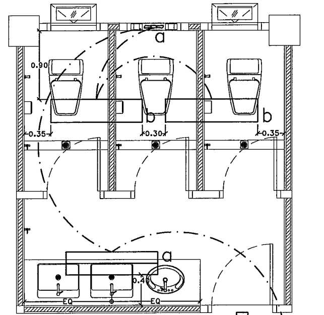
แปลนแสงสว่างห้องน้ำหญิงโรงเรียนลำอีต๊ะ ชั้นที่ 1-3 Scale 1 : 50
