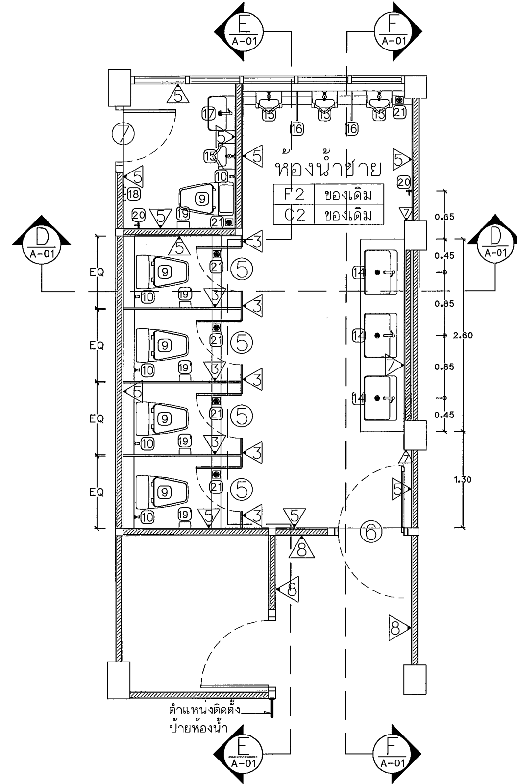
แปลนห้องน้ำชาย ชั้นที่ 2 และ 3 แบบปรับปรุง Scale 1 : 50
