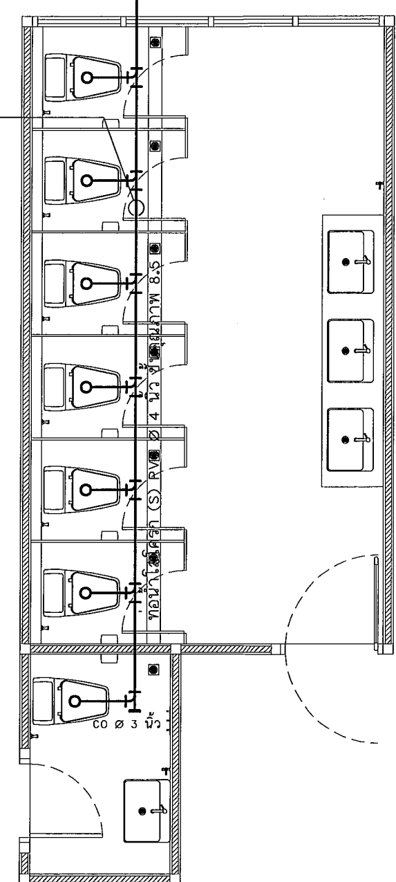
แปลนระบบน้ำโสโครกห้องน้ำหญิง ชั้นที่ 2 และ 3 Scale 1 : 50
