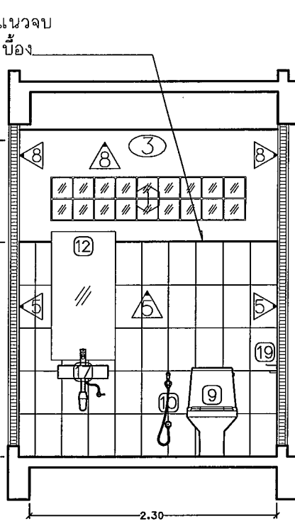
รูปตัดขยาย B Scale 1 : 50
