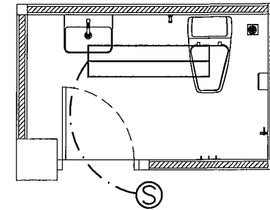
แปลนแสงสว่างห้องน้ำอาจารย์ ชั้นที่ 1, 2 และ 3 Scale 1 : 50
