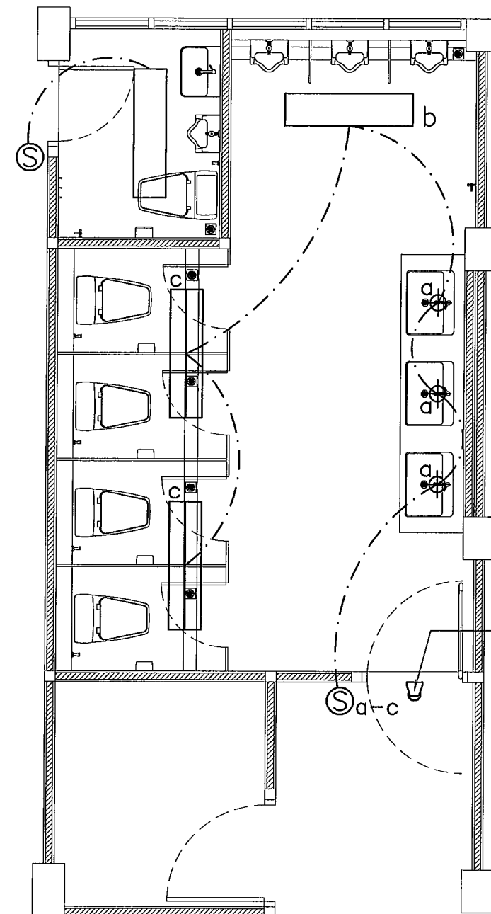
แปลนระบบไฟฟ้าแสงสว่างห้องน้ำชาย ชั้นที่ 2 และ 3 Scale 1 : 50
