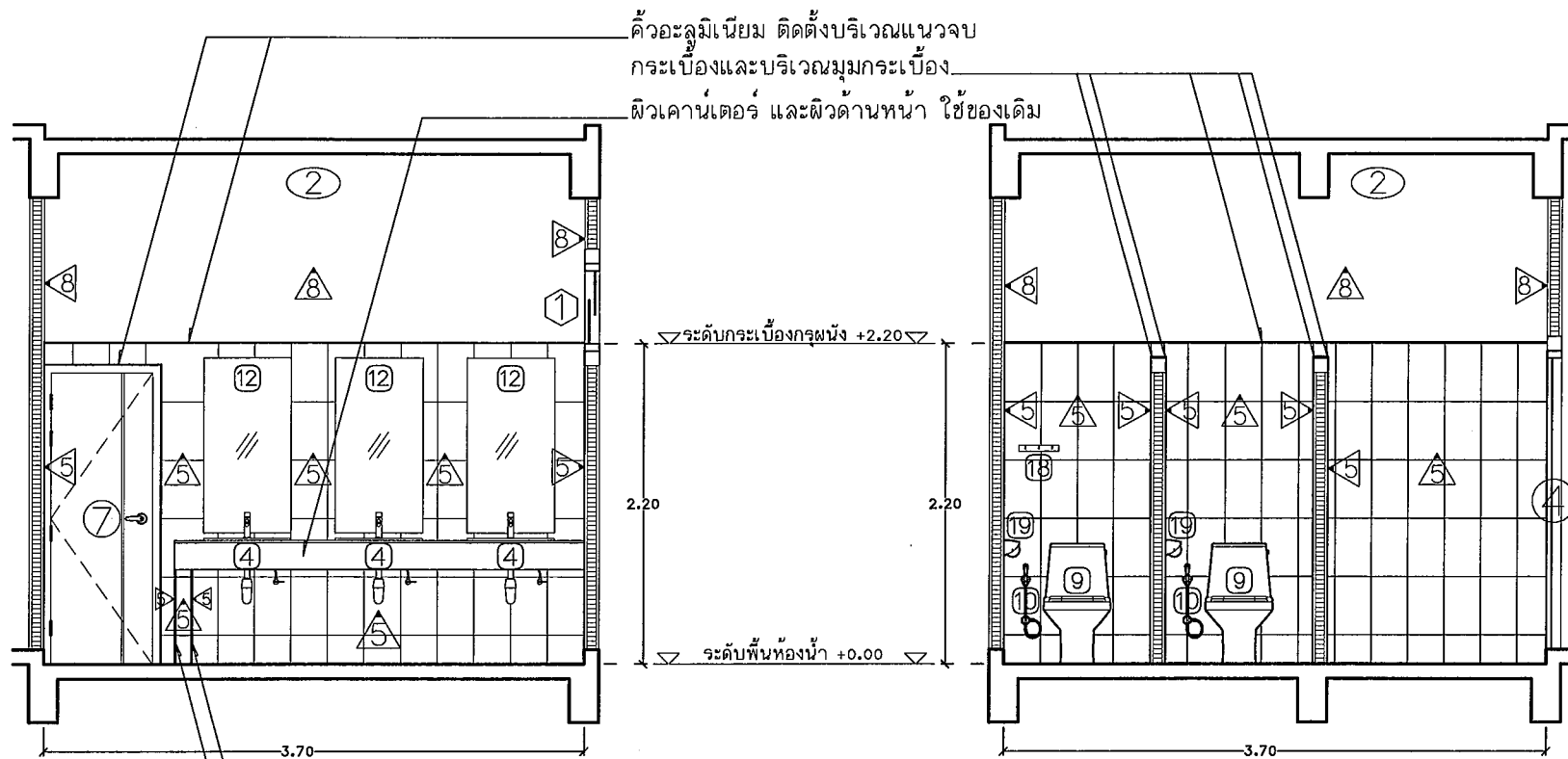
รูปตัดขยาย A Scale 1 : 50
