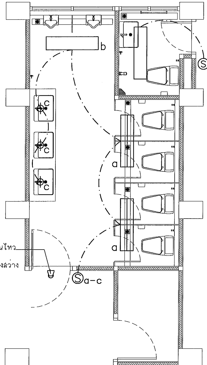
แปลนระบบไฟฟ้าแสงสว่างห้องน้ำชาย ชั้นที่ 2 Scale 1 : 50
