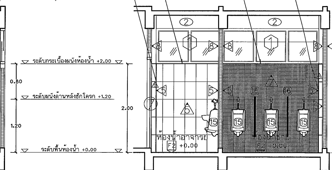
รูปตัดขยาย H Scale 1 : 50
