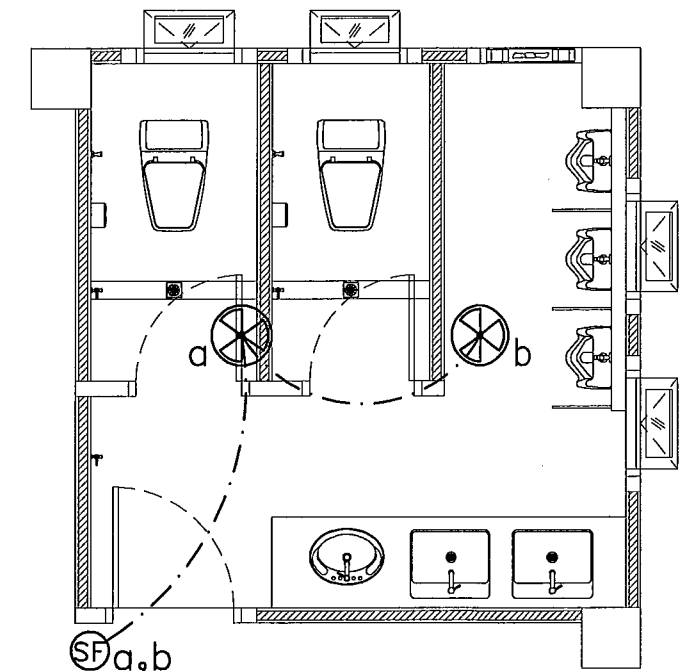
แปลนตำแหน่งพัดลมห้องน้ำชายโรงเรียนลำอีต๊ะ ชั้นที่ 1-3 Scale 1 : 50
