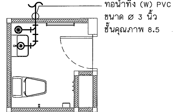
แปลนระบบน้ำทิ้งห้องน้ำอาจารย์ ชั้นที่ 1 Scale 1 : 50
