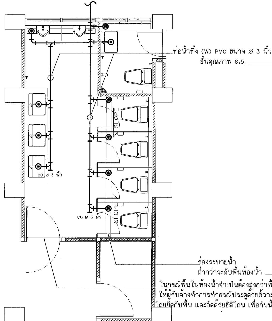
แปลนระบบน้ำทิ้งห้องน้ำอาจารย์ ชั้นที่ 1 Scale 1 : 50
