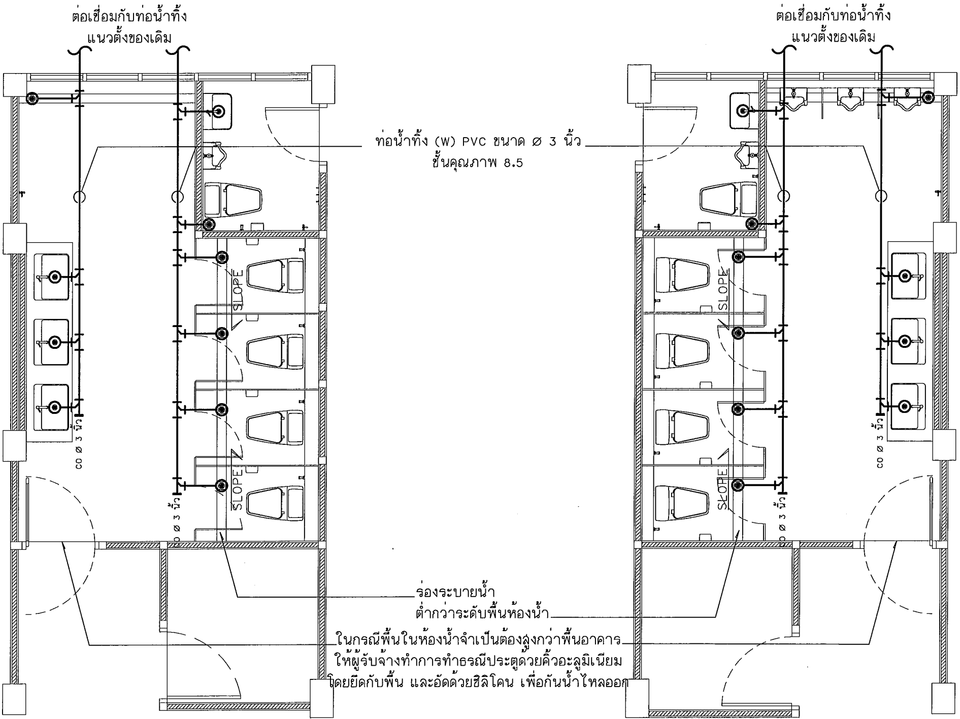
แปลนระบบน้ำทิ้งห้องน้ำหญิง ชั้นที่ 2 และ 3 Scale 1 : 50
