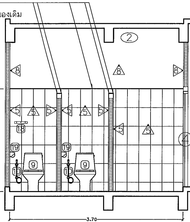
รูปตัดขยาย B Scale 1 : 50
