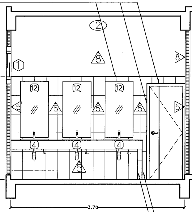
รูปตัดขยาย G Scale 1 : 50
