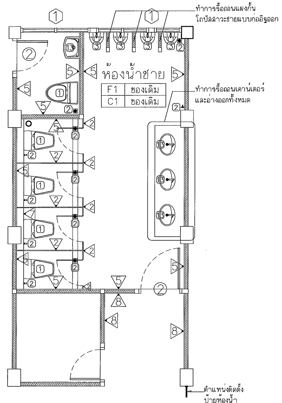
แปลนห้องน้ำชาย ชั้นที่ 2 เดิม Scale 1 : 50
