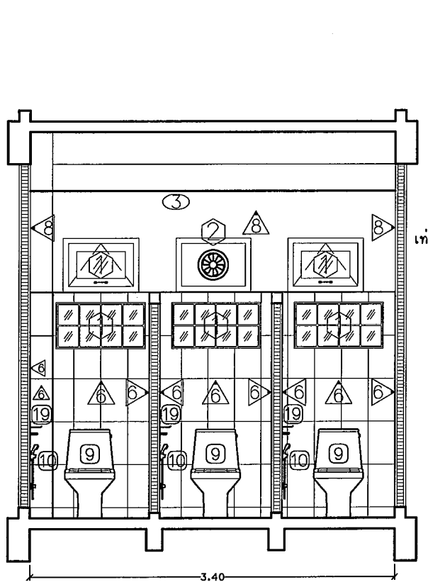
รูปตัดขยาย A Scale 1 : 50
