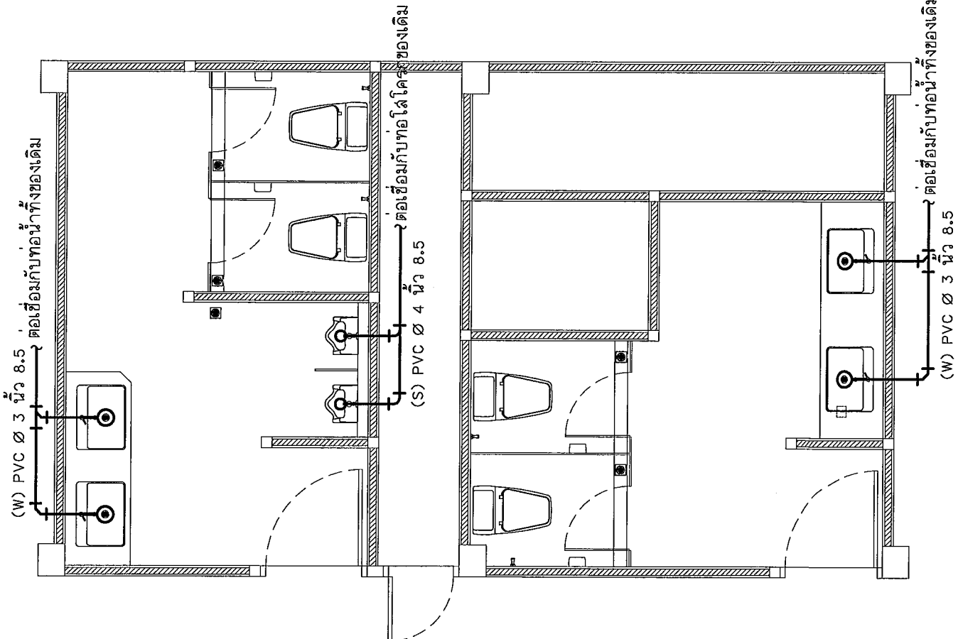
แปลนระบบน้ำทิ้ง และน้ำใส่โครก ห้องน้ำห้องประชุมควาลัย Scale 1 : 50
