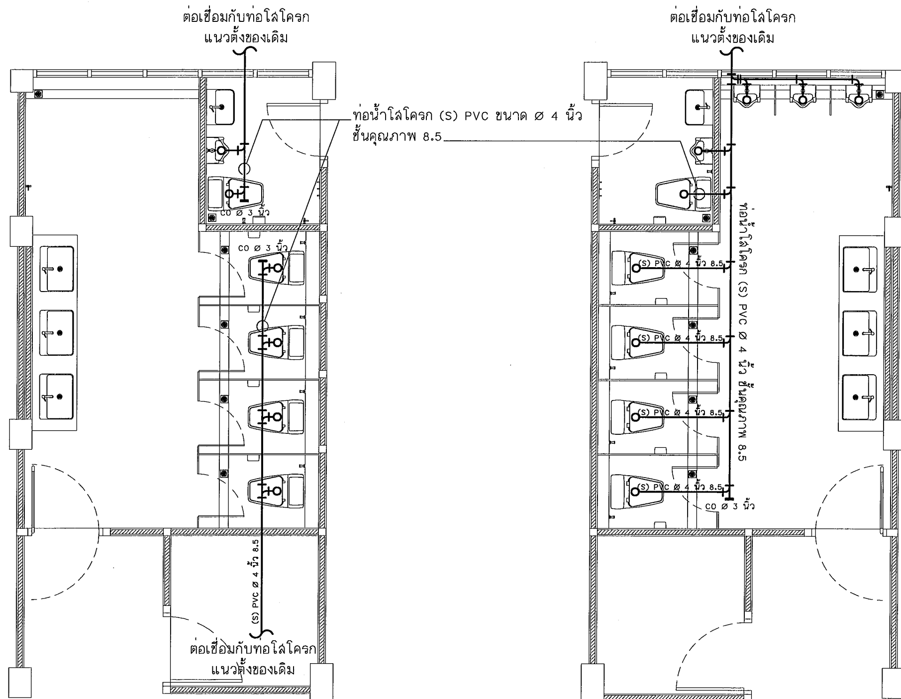
แปลนระบบน้ำไลโครกห้องน้ำหญิง ชั้นที่ 2 และ 3
