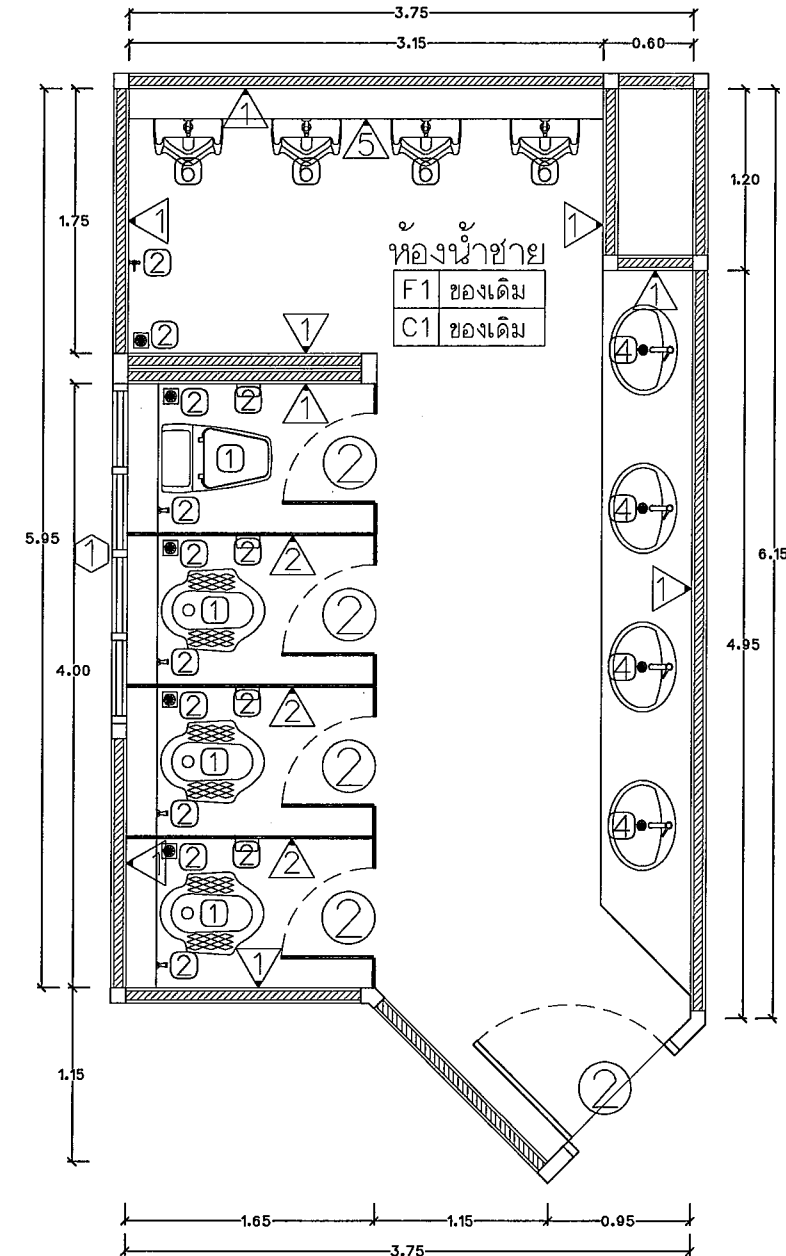
แปลนห้องน้ำชาย ชั้นที่ 1-9 เดิม Scale 1 : 50
