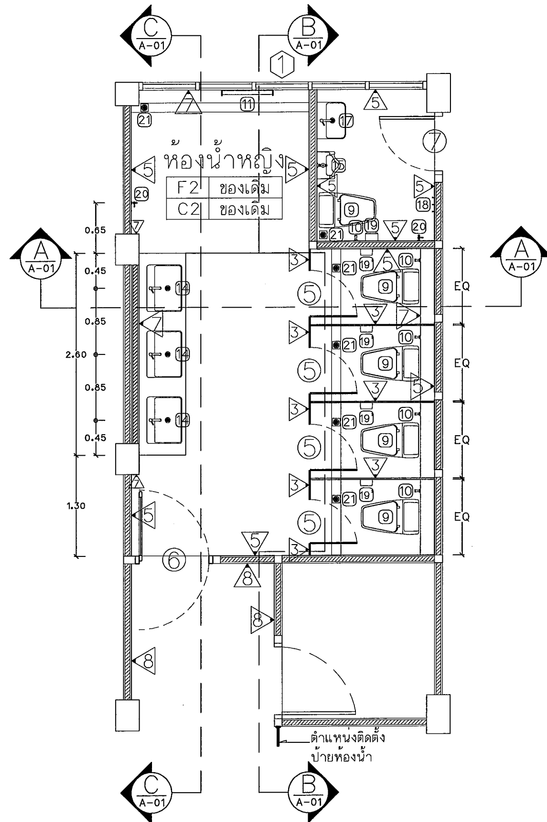
แปลนห้องน้ำหญิง ชั้นที่ 2 และ 3 แบบปรับปรุง Scale 1 : 50
