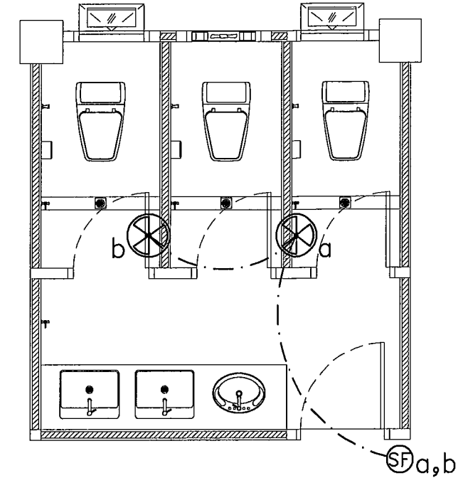
แปลนตำแหน่งพัดลมห้องน้ำหญิงโรงเรียนลำอีต๊ะ ชั้นที่ 1-3 Scale 1 : 50
