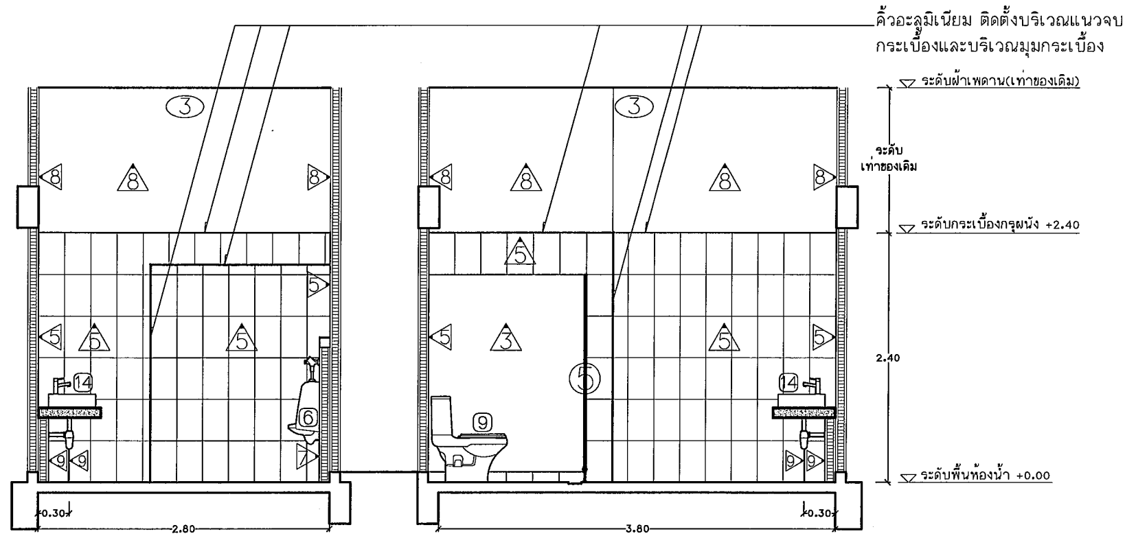
รูปตัดขยาย A Scale 1 : 50
