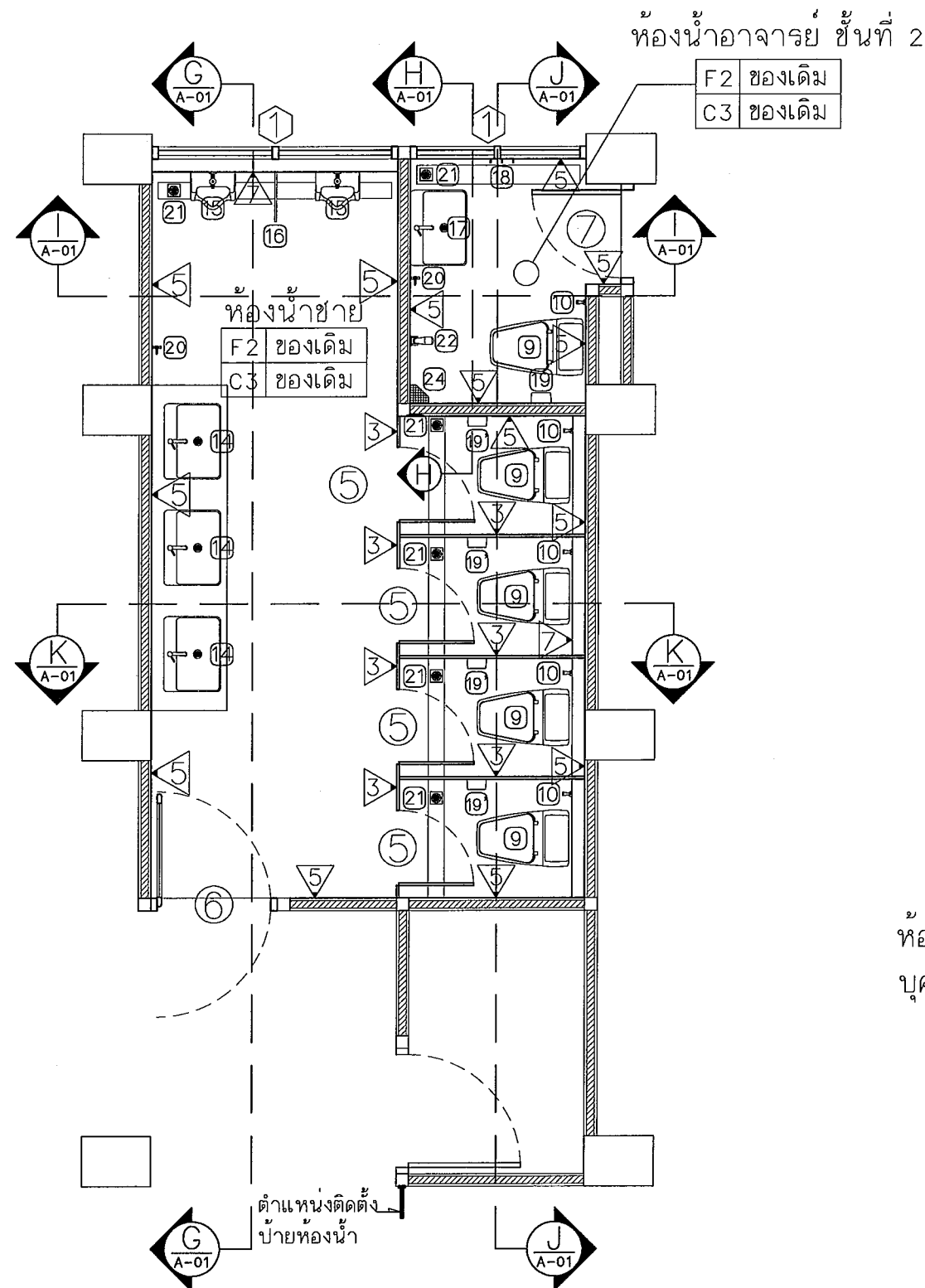
แปลนห้องน้ำชาย ชั้นที่ 2 แบบปรับปรุง
