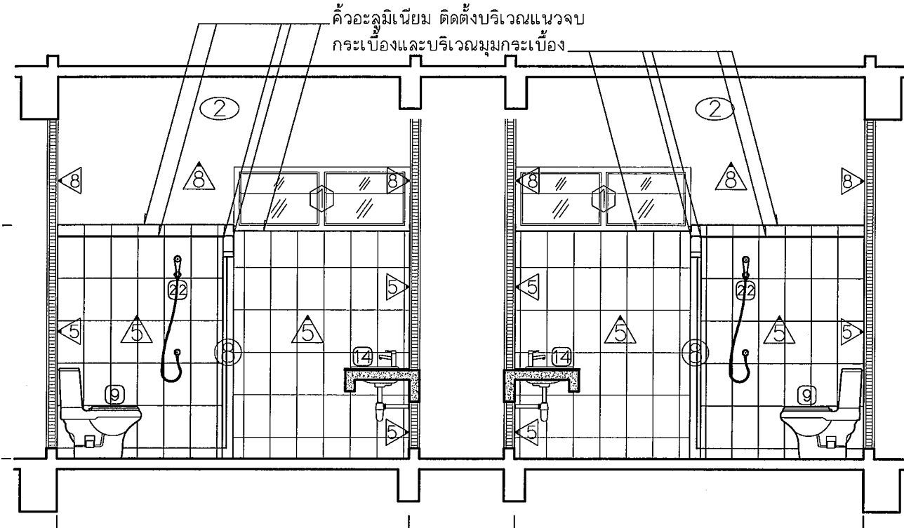
รูปตัดขยาย J Scale 1 : 50
