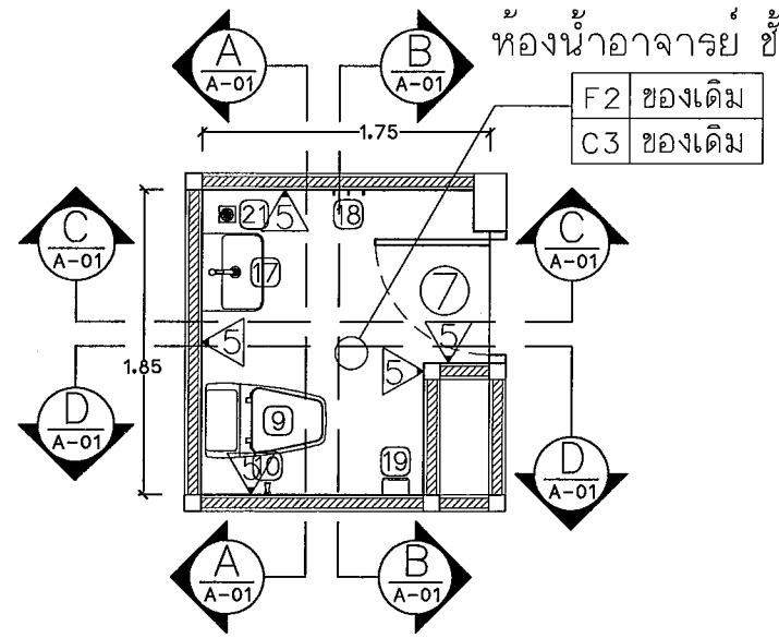
แปลนห้องน้ำอาจารย์ ชั้นที่ 1 ของใหม่ Scale 1 : 50
