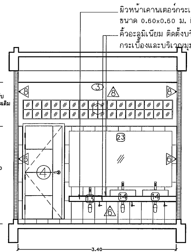
รูปตัดขยาย B Scale 1 : 50
