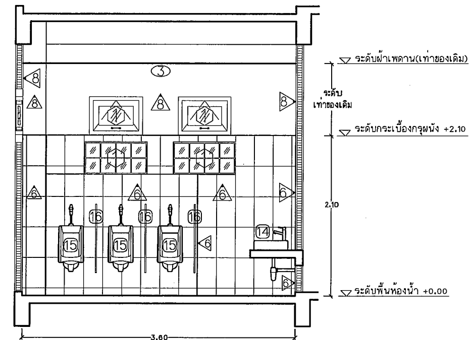
รูปตัดขยาย F Scale 1 : 50
