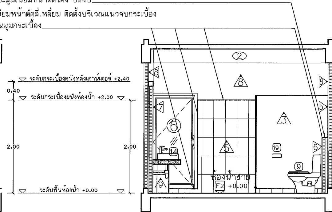
รูปตัดขยาย F Scale 1 : 50
