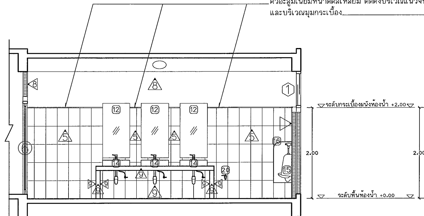
รูปตัดขยาย G Scale 1 : 50
