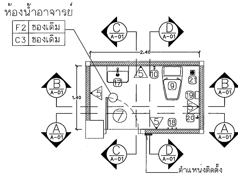
แปลนห้องน้ำอาจารย์ ชั้นที่ 1, 2 และ 3 แบบปรับปรุง Scale 1 : 50
