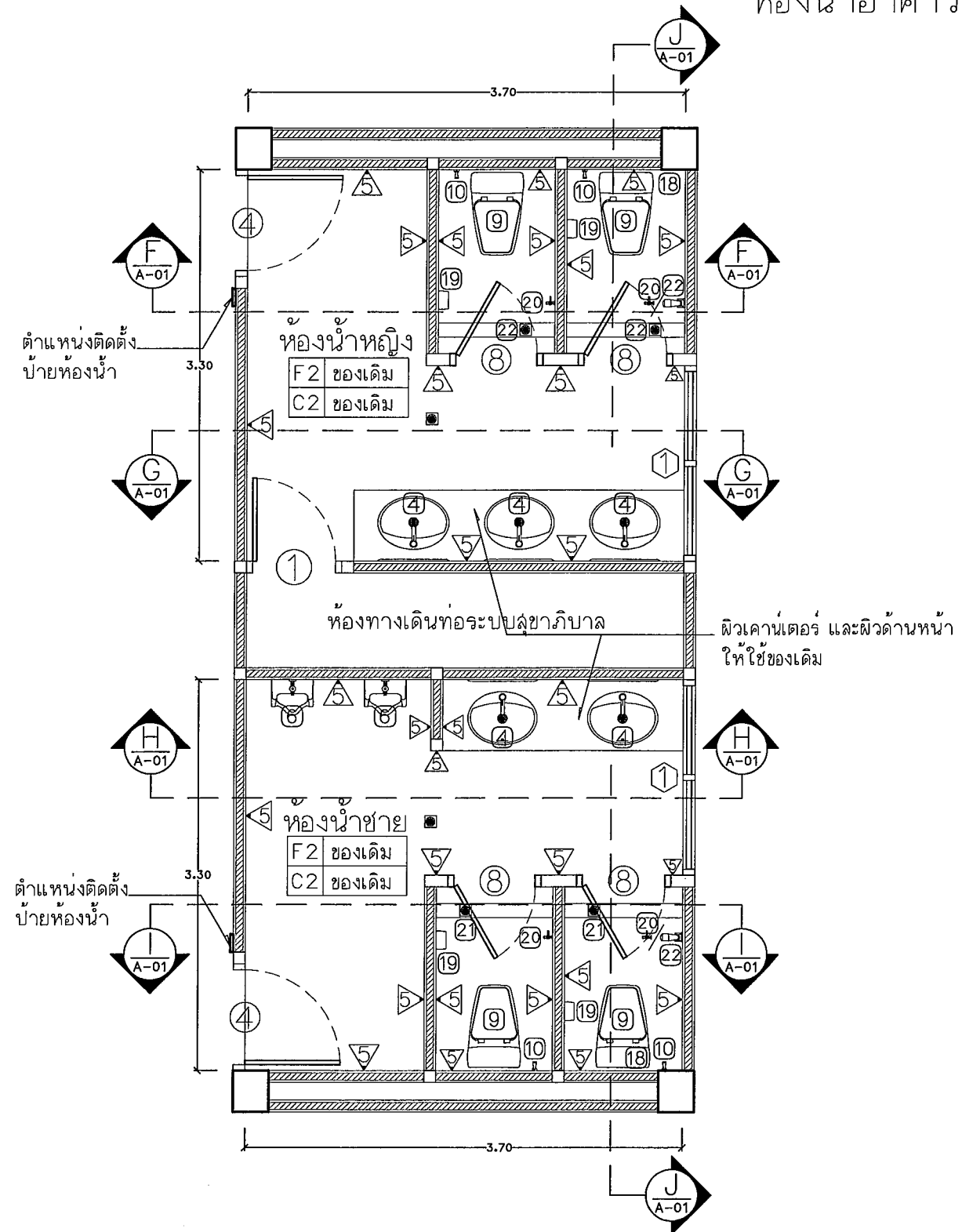
แปลนห้องน้ำชาย-หญิงชั้น 2 และ 3 (ทิศใต้) แบบปรับปรุง Scale 1 : 50
