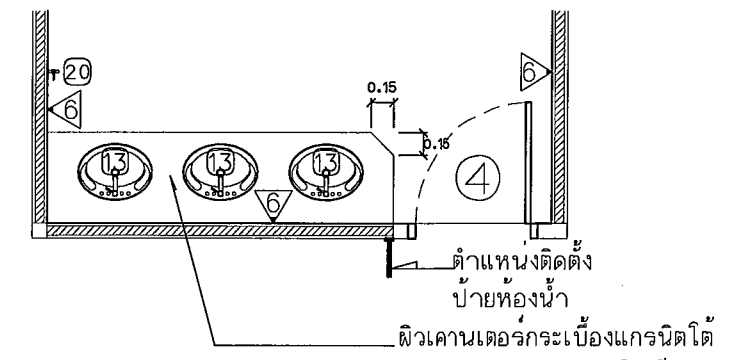
แปลนห้องน้ำหญิงโรงเรียนลำอิตฯ ชั้นที่ 3 แบบปรับปรุง Scale 1 : 50
