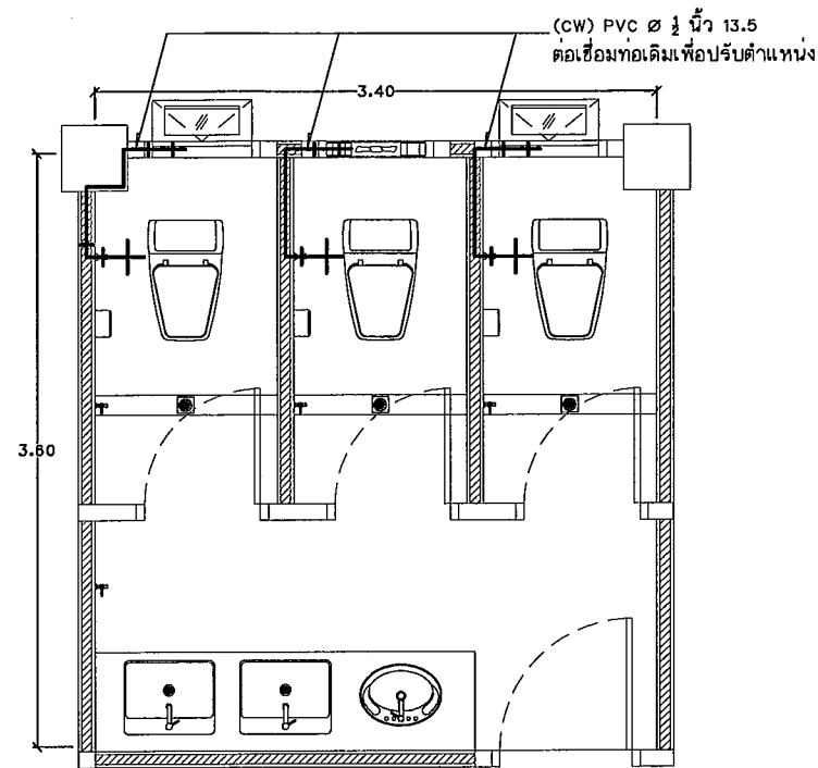
แปลนระบบน้ำดีห้องน้ำหญิงโรงเรียนลำอีต๊ะ ชั้นที่ 1-3 Scale 1 : 50
