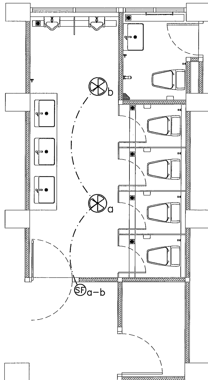
แปลนตำแหน่งพัฒมห้องน้ำชาย ชั้นที่ 2 Scale 1 : 50
