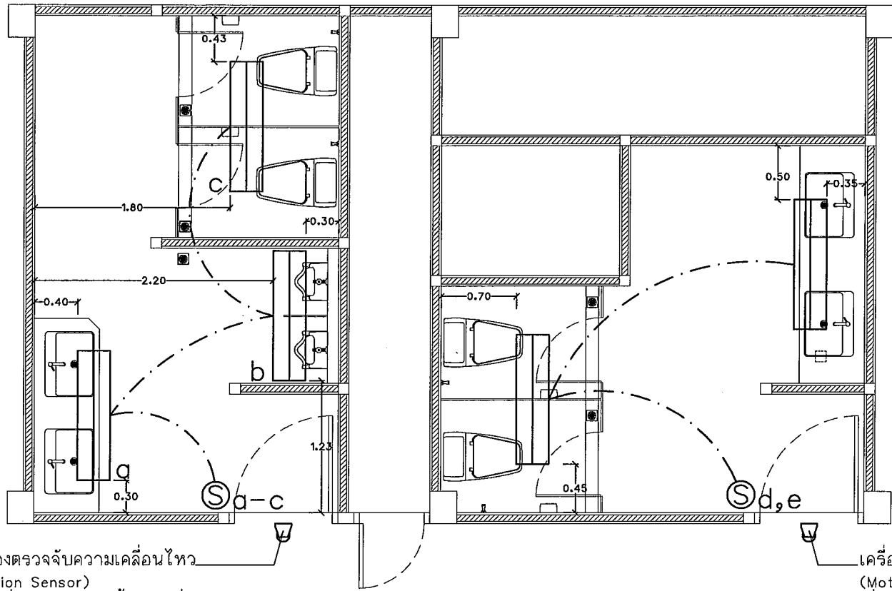
แปลนแสงสว่าง ห้องน้ำห้องประชุมควิลัย Scale 1 : 50
