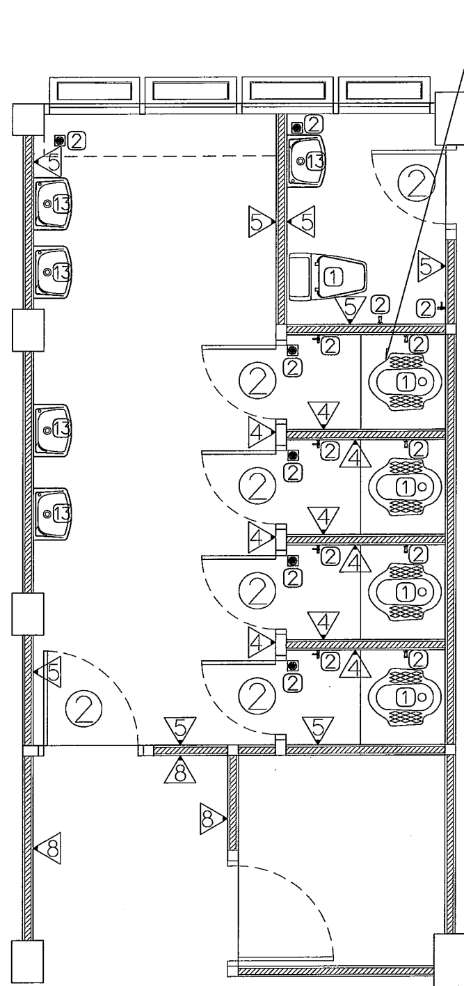
แปลนห้องน้ำหญิง ชั้นที่ 2 และ 3 เดิม Scale 1 : 50
