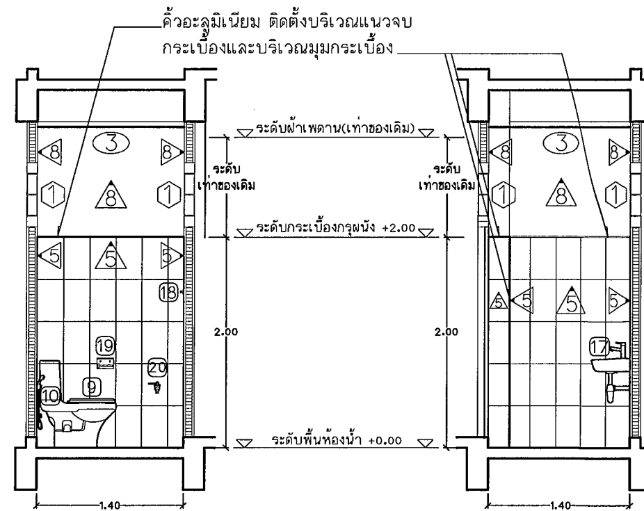
รูปตัดขยาย C Scale 1 : 50
