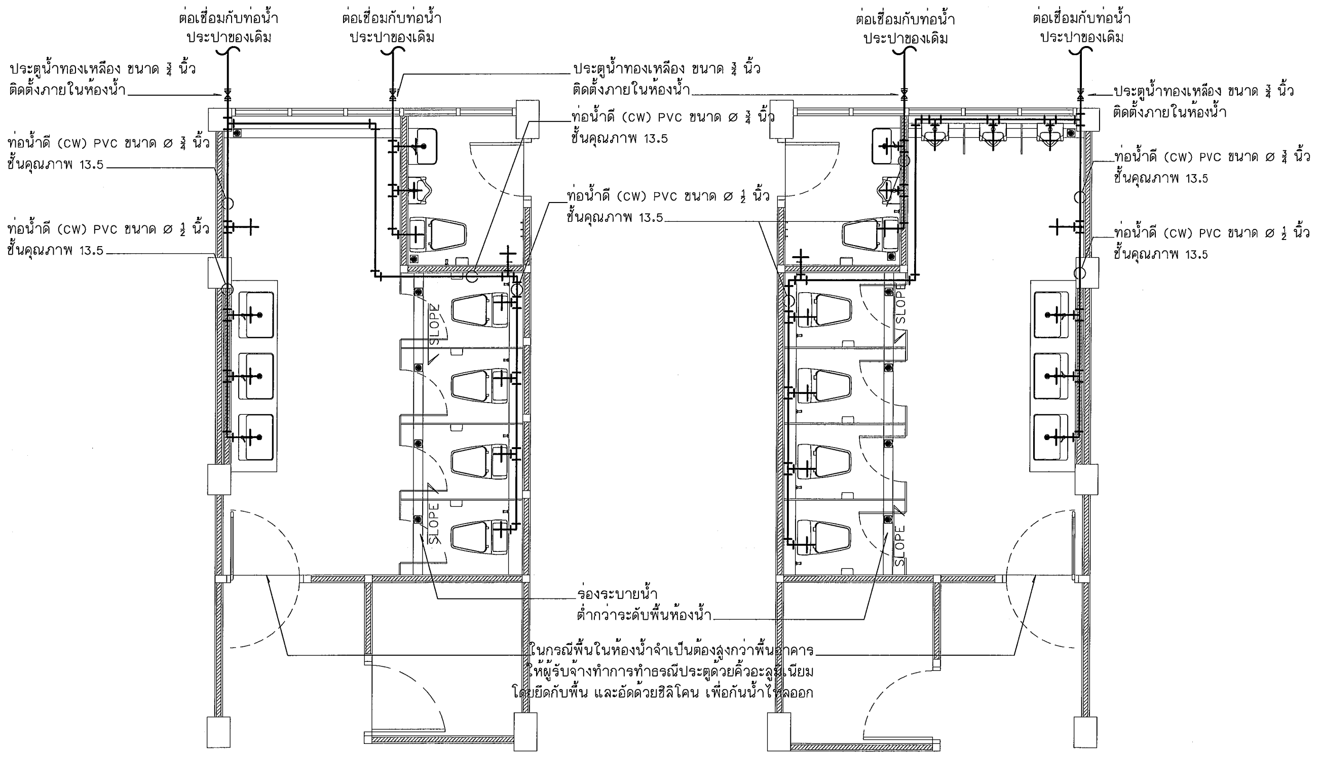
แปลนระบบน้ำดีห้องน้ำหญิง ชั้นที่ 2 และ 3 Scale 1 : 50
