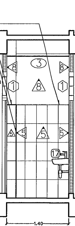
รูปตัดขยาย D Scale 1 : 50
