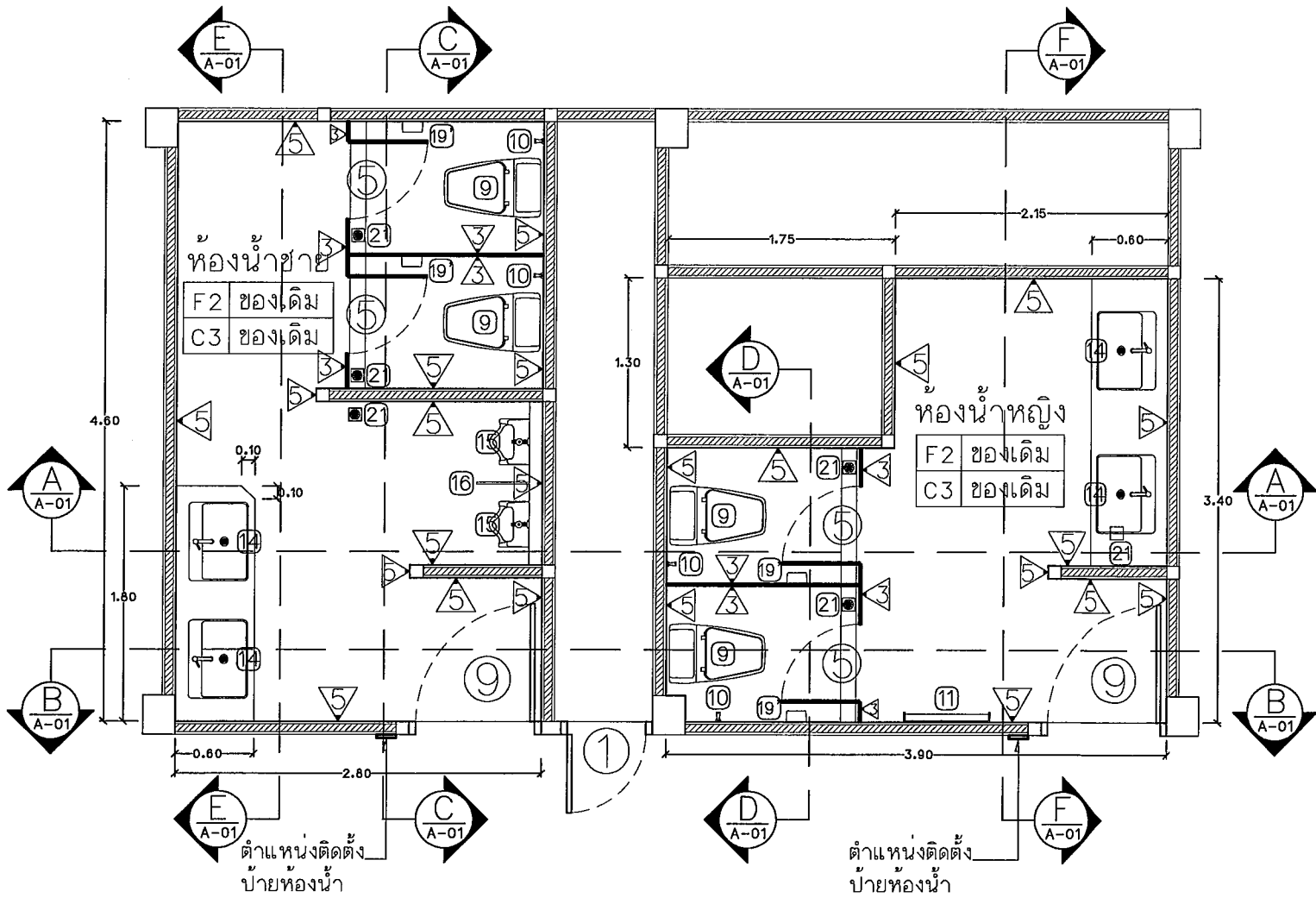
แปลนห้องน้ำชาย - หญิง ห้องประชุมคิวลัย แบบปรับปรุง Scale 1 : 50
