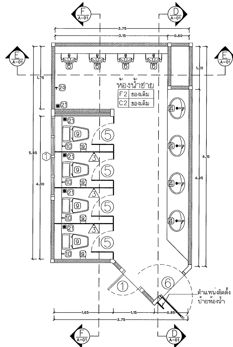
แปลนห้องน้ำชายชั้นที่ 1-9 แบบปรับปรุง Scale 1 : 50
