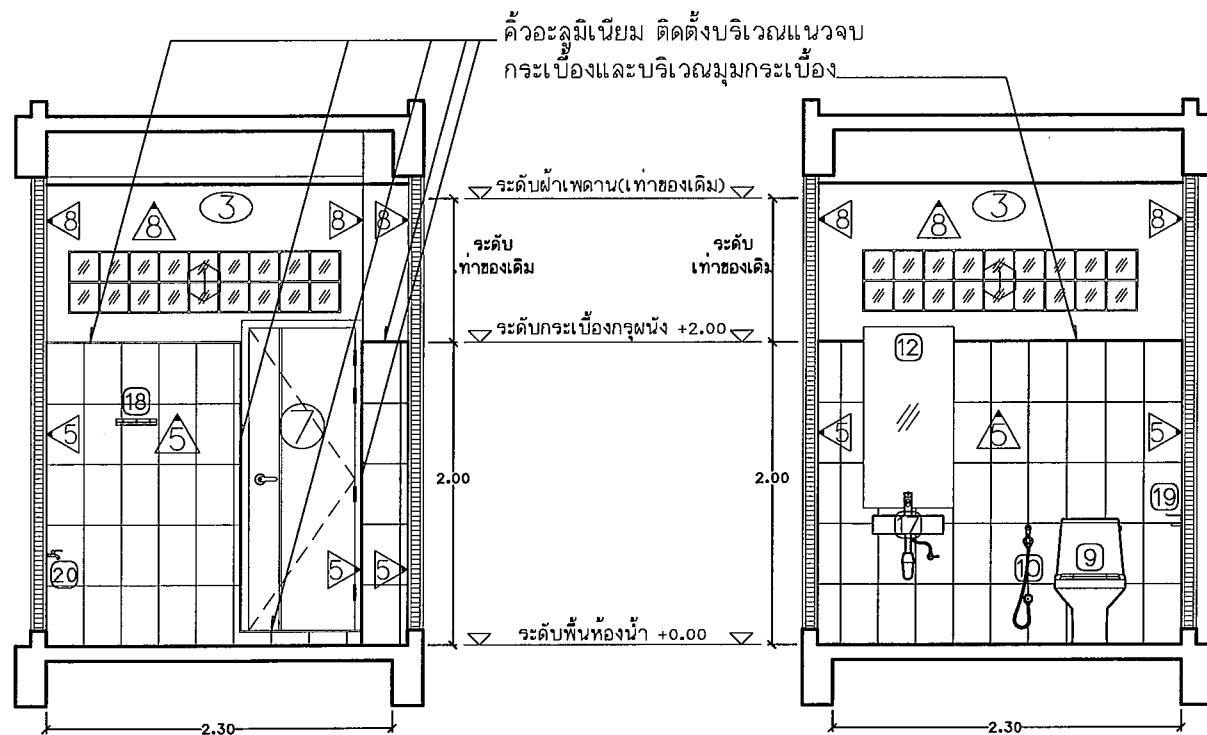
รูปตัดขยาย A Scale 1 : 50
