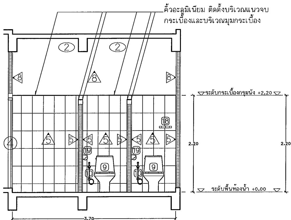
รูปตัดขยาย D Scale 1 : 50
