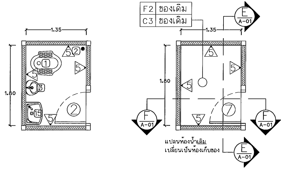
แปลนห้องน้ำเดิมผังตะวันตก ชั้นที่ 1 Scale 1 : 50
