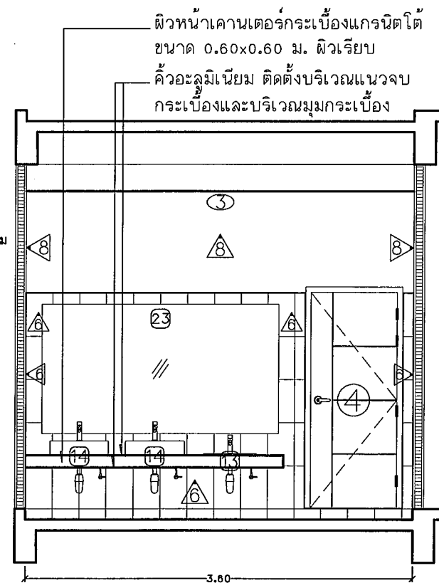
รูปตัดขยาย E Scale 1 : 50
