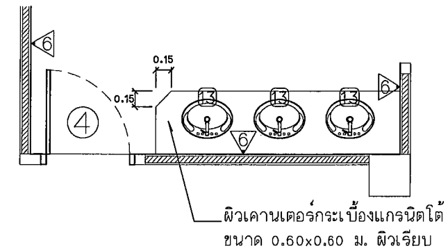
แปลนห้องน้ำชายโรงเรียนลำอิตา ชั้นที่ 3 แบบปรับปรุง Scale 1 : 50
