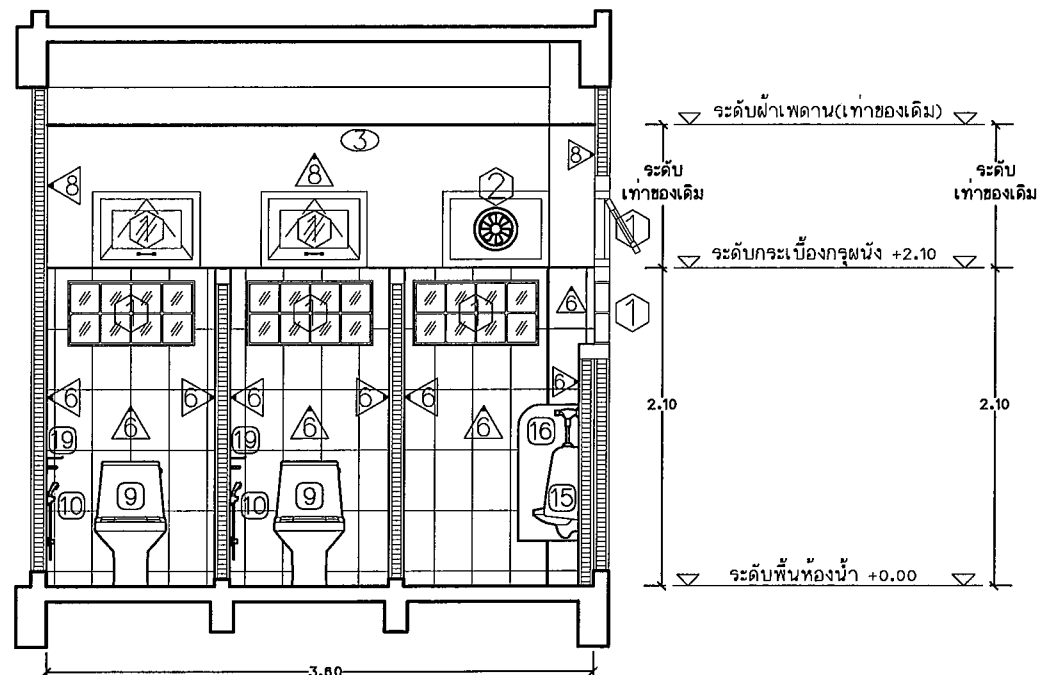
รูปตัดขยาย D Scale 1 : 50
