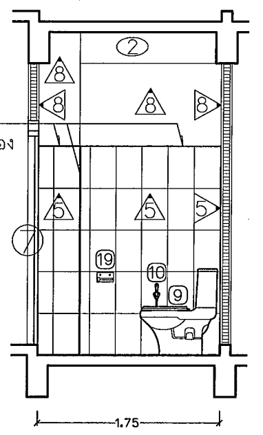
รูปตัด D Scale 1 : 50
