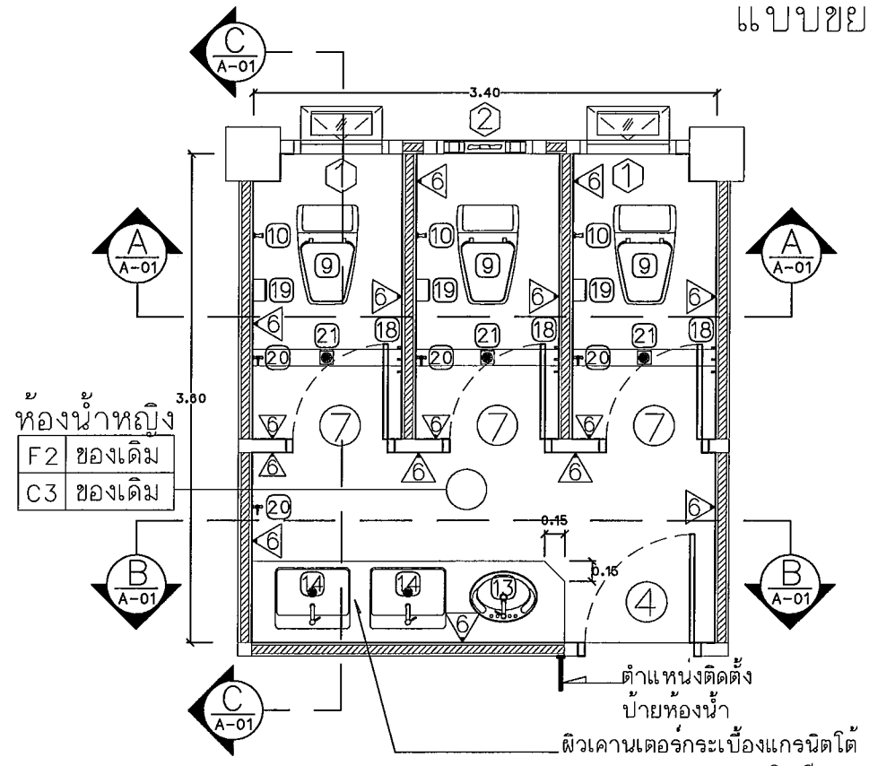
แปลนห้องน้ำหญิงโรงเรียนลำอิตฯ ชั้นที่ 1-2 แบบปรับปรุง Scale 1 : 50
