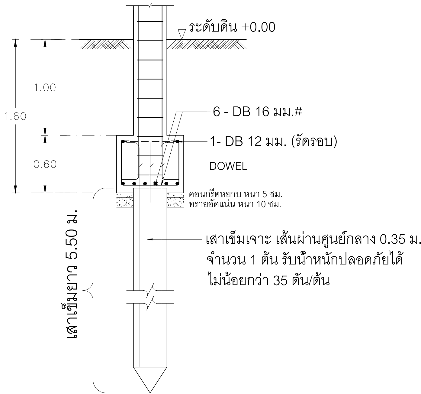
ขยายรูปตัด A มาตราส่วน 1:25
