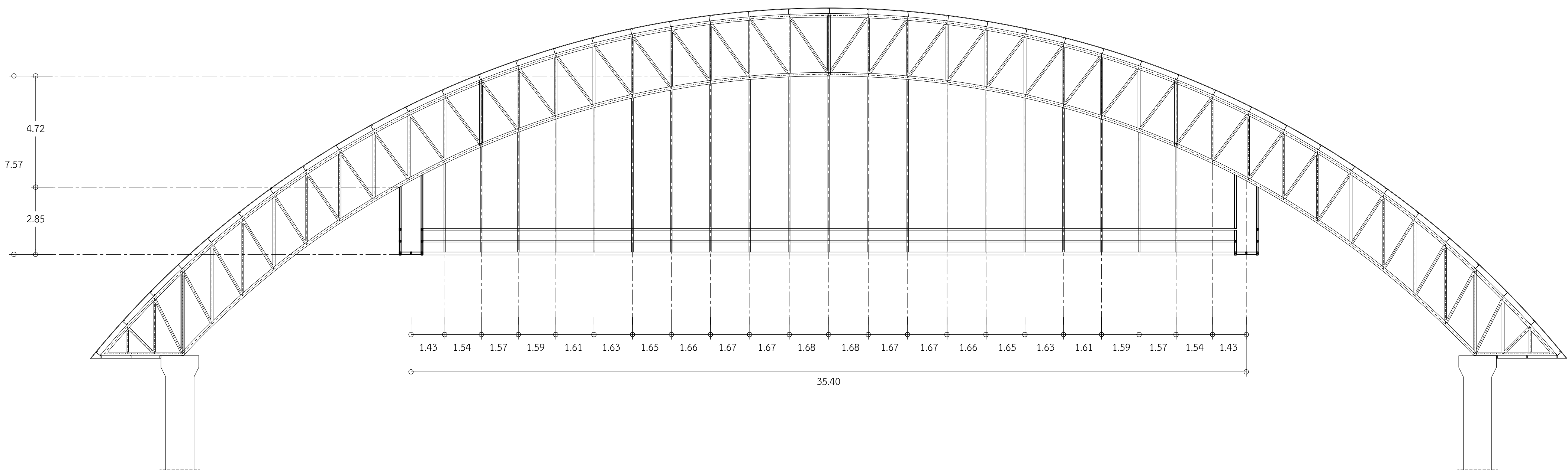
แบบ CATWALK
