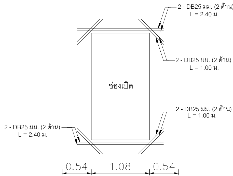
เหล็กเสริมช่องเปิด
