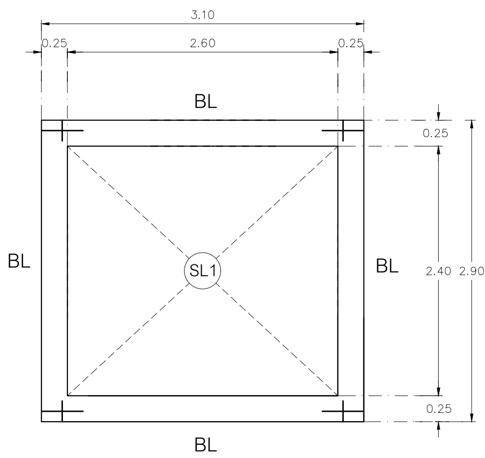
แปลนหลังคาห้องเครื่องลิฟท์ มาตราส่วน 1 : 25
