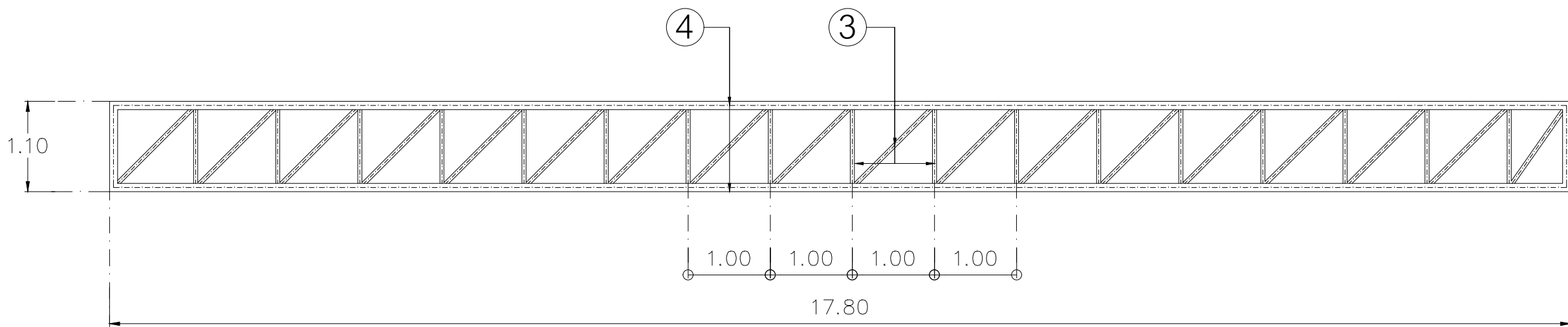
แบบขยาย T-12
