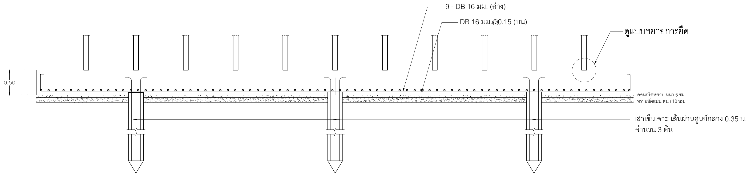
ขยายรูปตัด A มาตราส่วน 1:25
