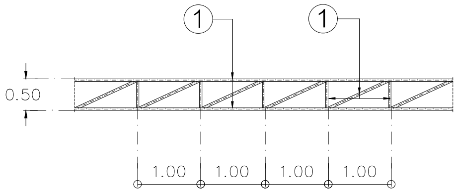
แบบขยาย T-11
