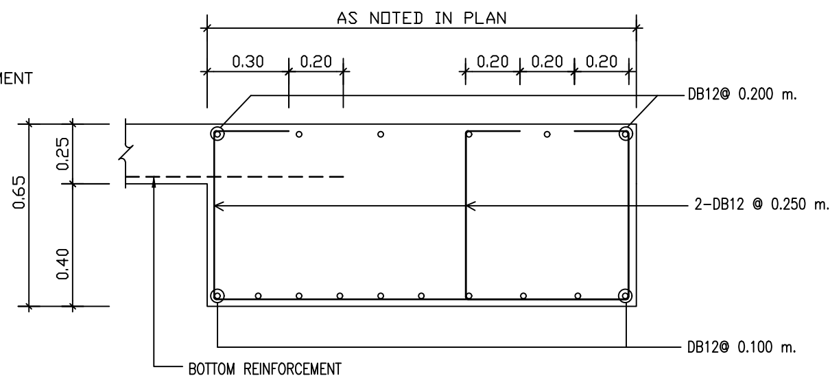
PB3 0.65 M.THK. (L-SHAPE)
