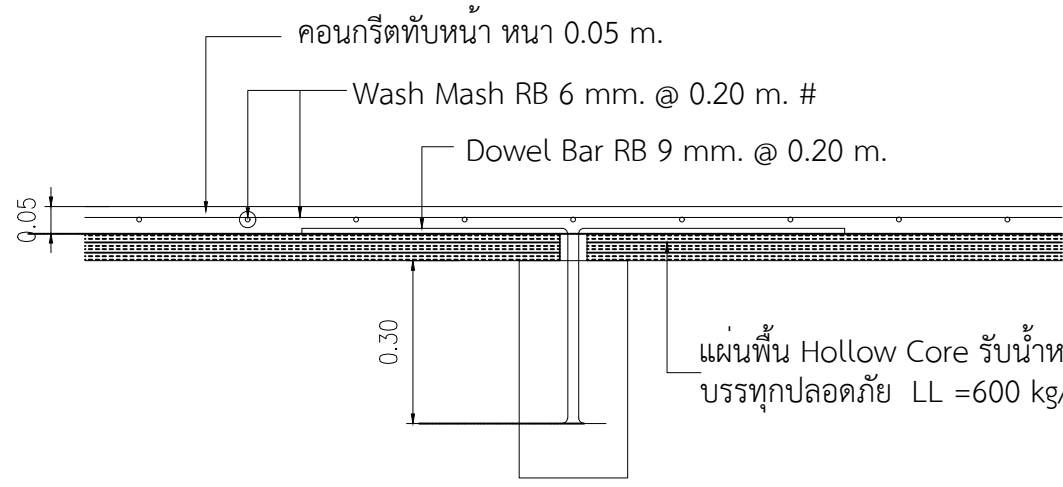
ขยายพื้น HC2
