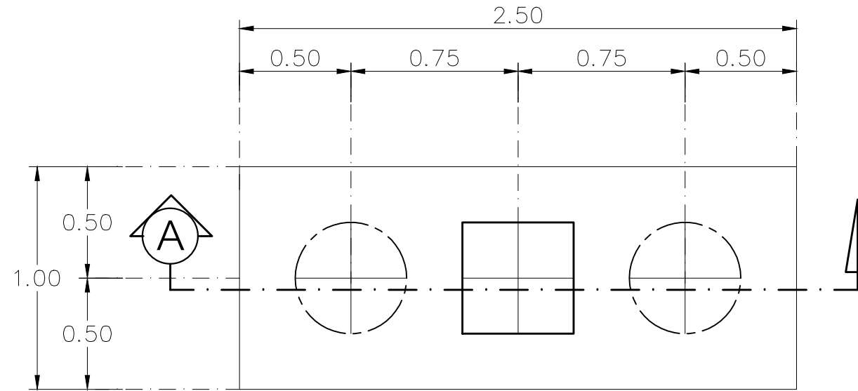
ขยายแปลนฐานราก F2 มาตราส่วน 1:25
