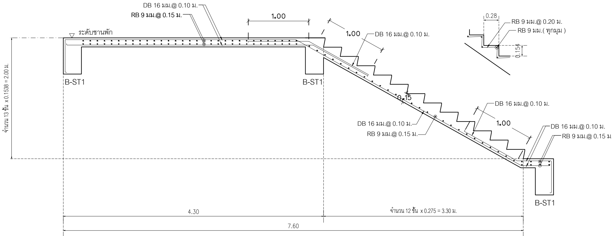
ST-1 ( พื้น - ขานพัก ) (บันไดหลัก)
