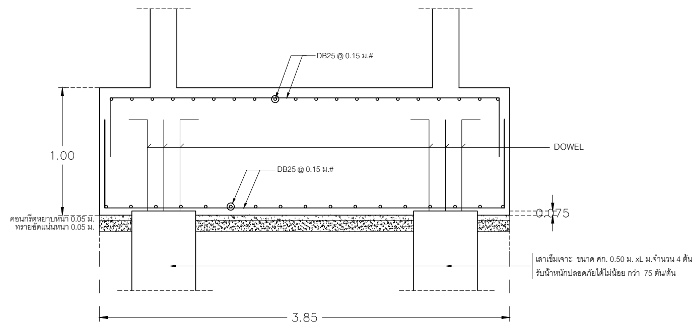
รูปตัด A
