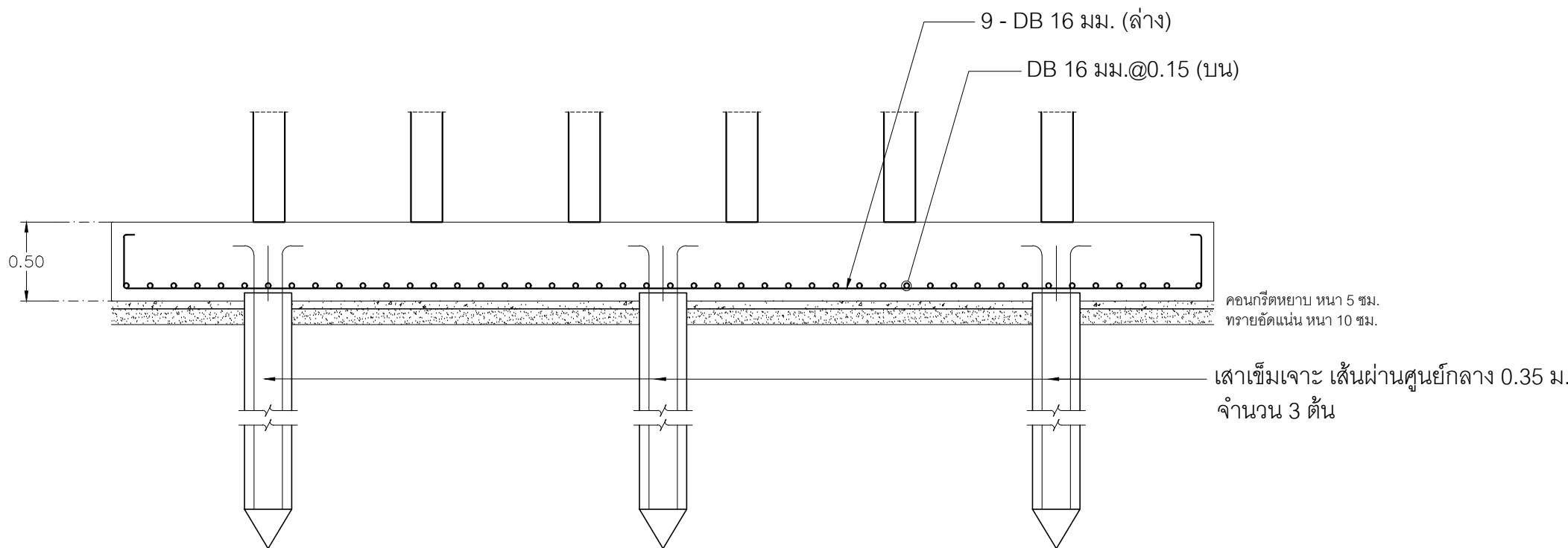
ขยายรูปตัด A มาตราส่วน 1:25
