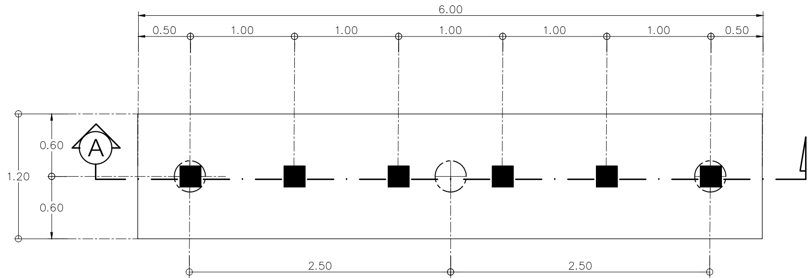
ขยายแปลนฐานราก FX1 มาตราส่วน 1:25
