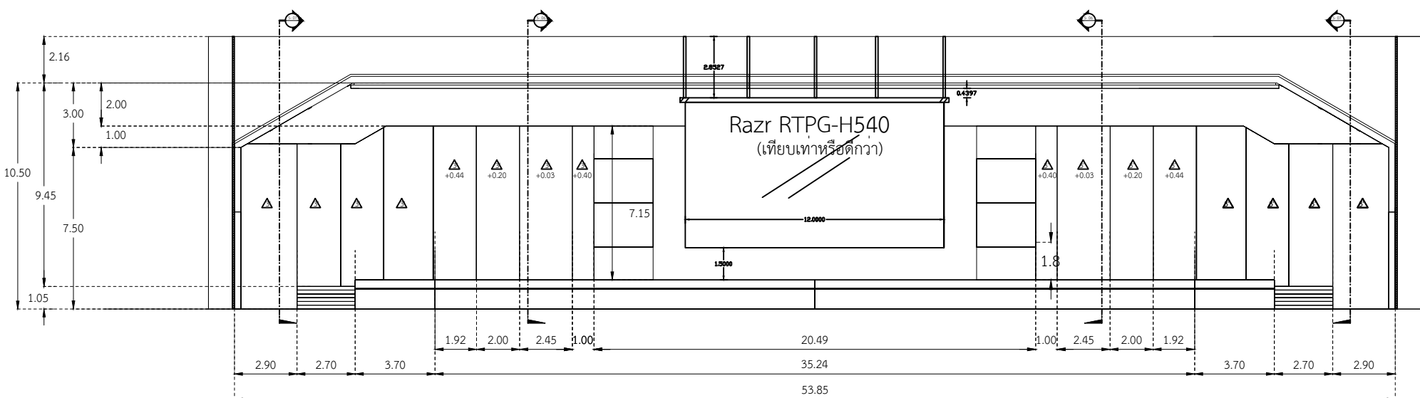
รูปด้าน B (หน้าฉากเวที) มาตราส่วน 1 : 200
