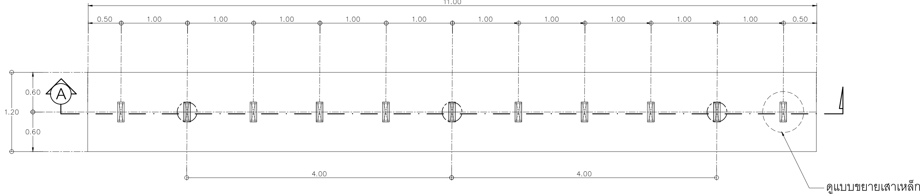
ขยายแปลนฐานราก FX2 มาตราส่วน 1:25
