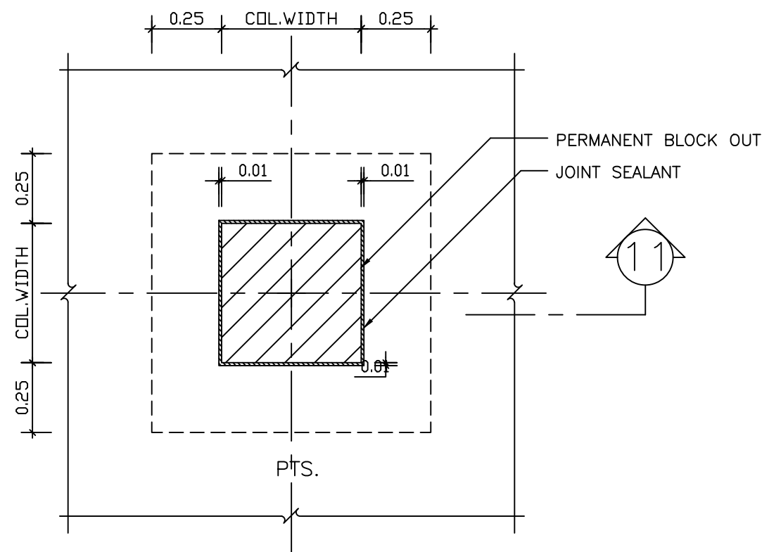
CORBEL PLAN (กรณี BLOCK OUT เล็กๆ) (INTERIOR COLUMN)
