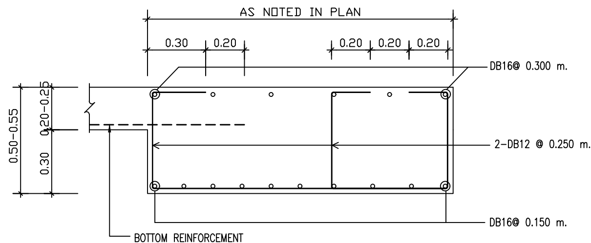
PB2 0.50-0.55 M.THK. (L-SHAPE)
