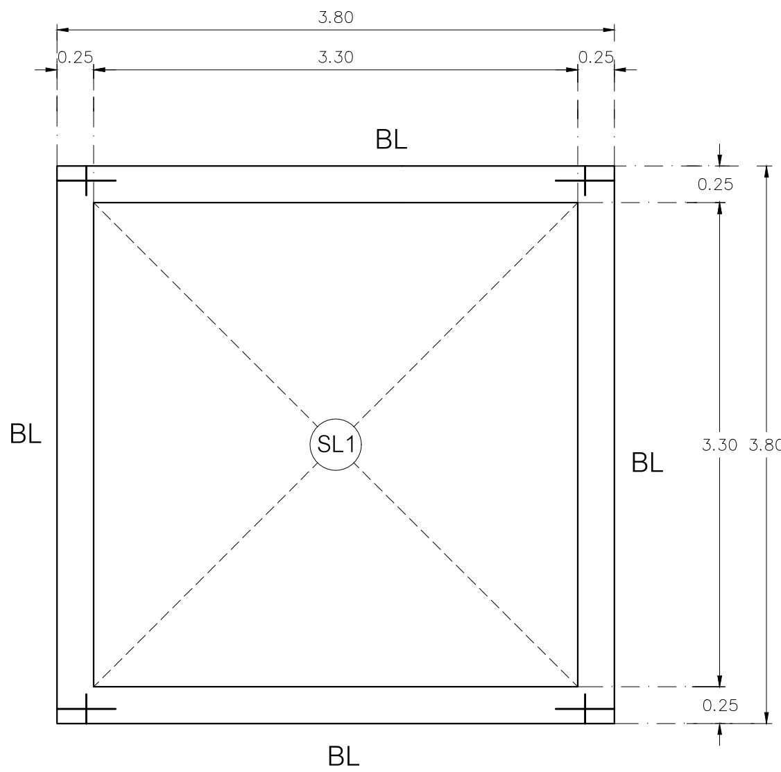
แปลนหลังคาห้องเครื่องลิฟท์ มาตราส่วน 1 : 25
