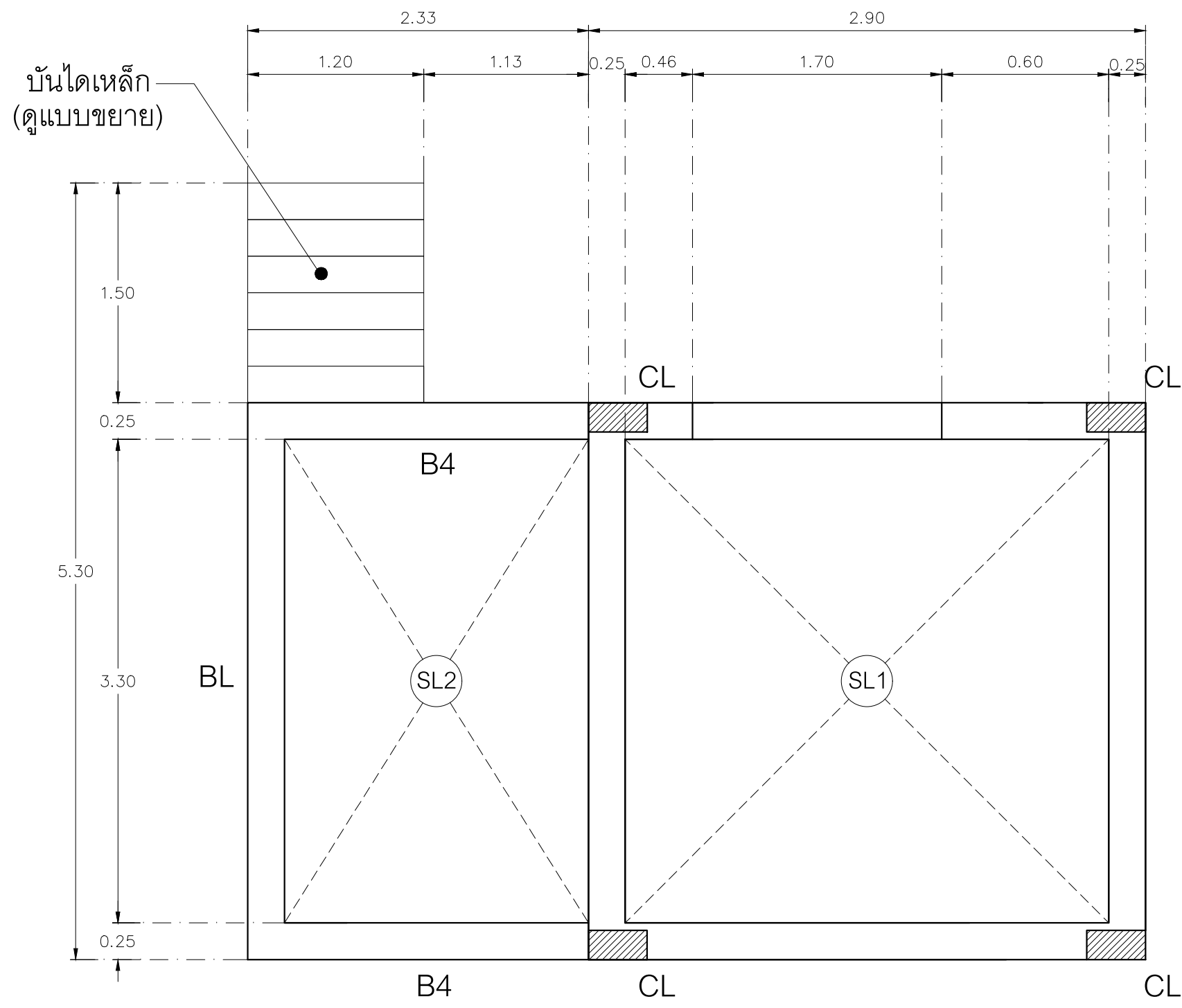
แปลนคานห้องเครื่องลิฟท์ มาตราส่วน
