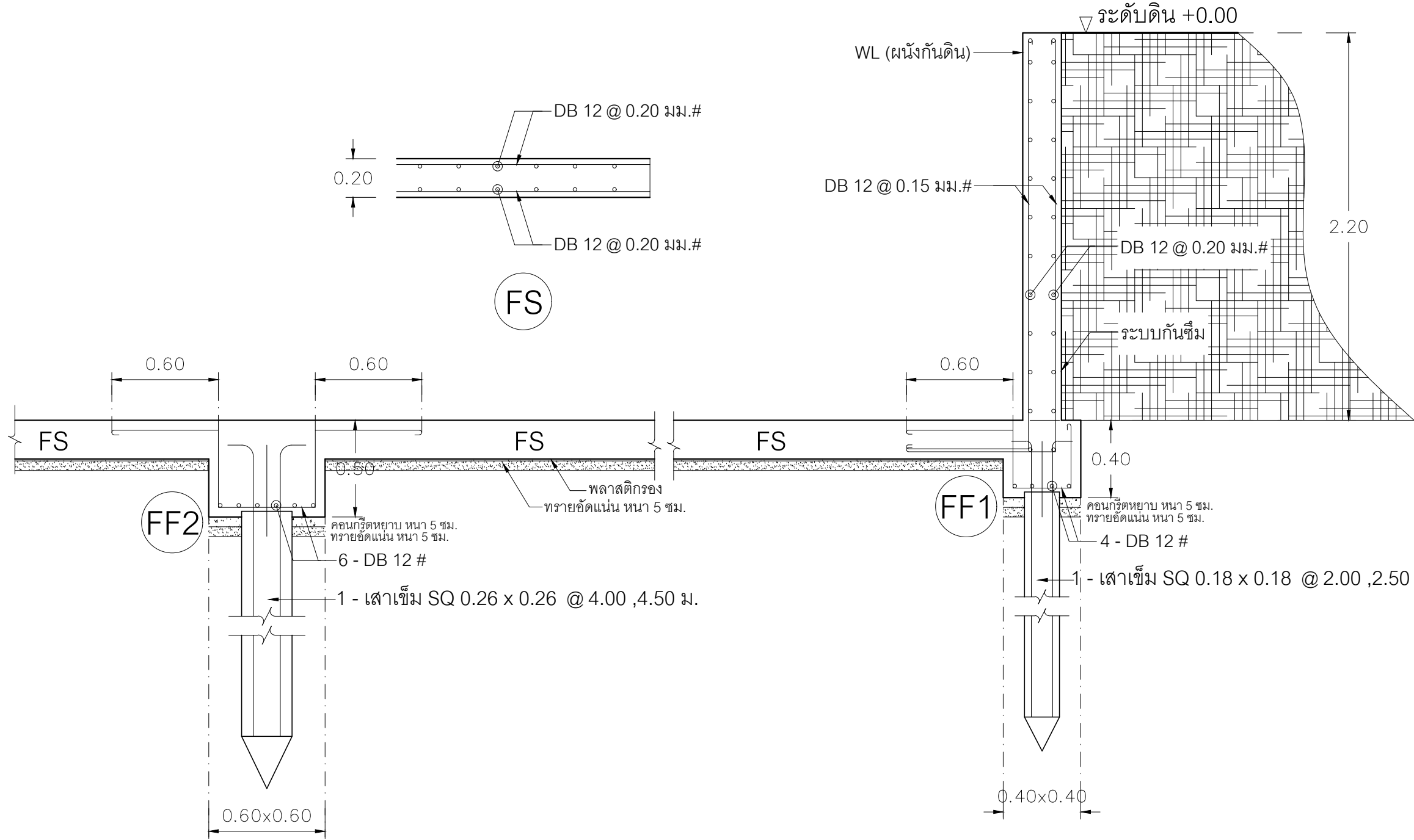
ขยายพื้น FS และผนังกันดิน WL มาตราส่วน 1:25
