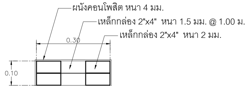
ขยายแปลน
