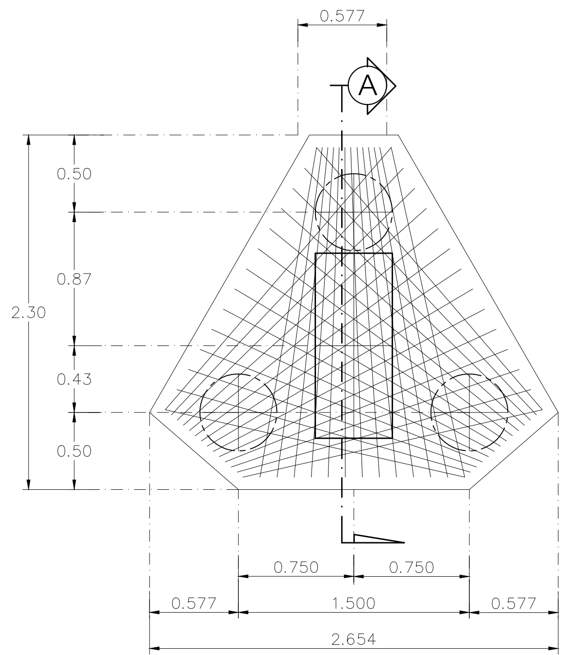
ขยายแปลนฐานราก F3 มาตราส่วน 1:25
