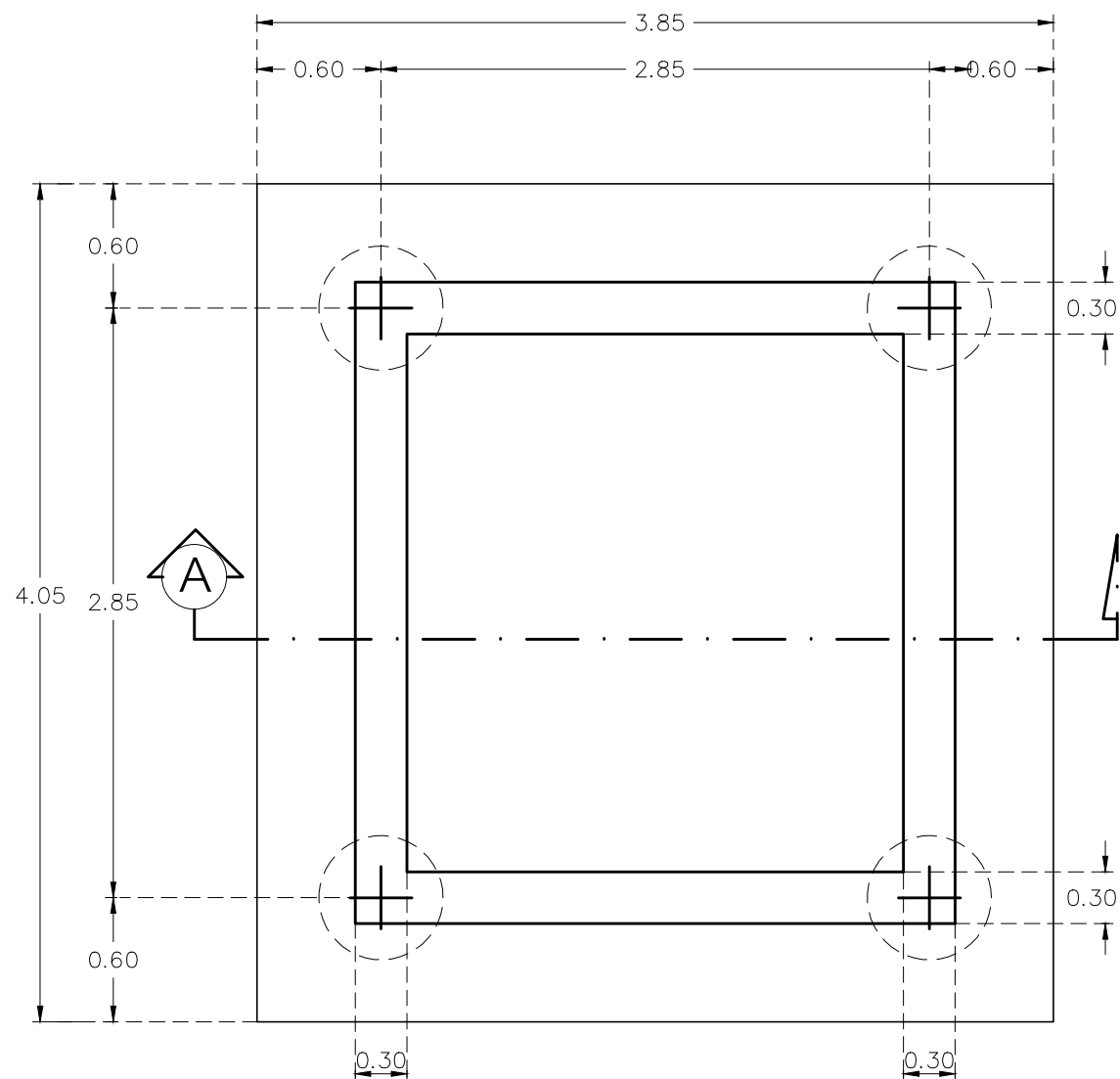
แปลน(ฐานราก)
