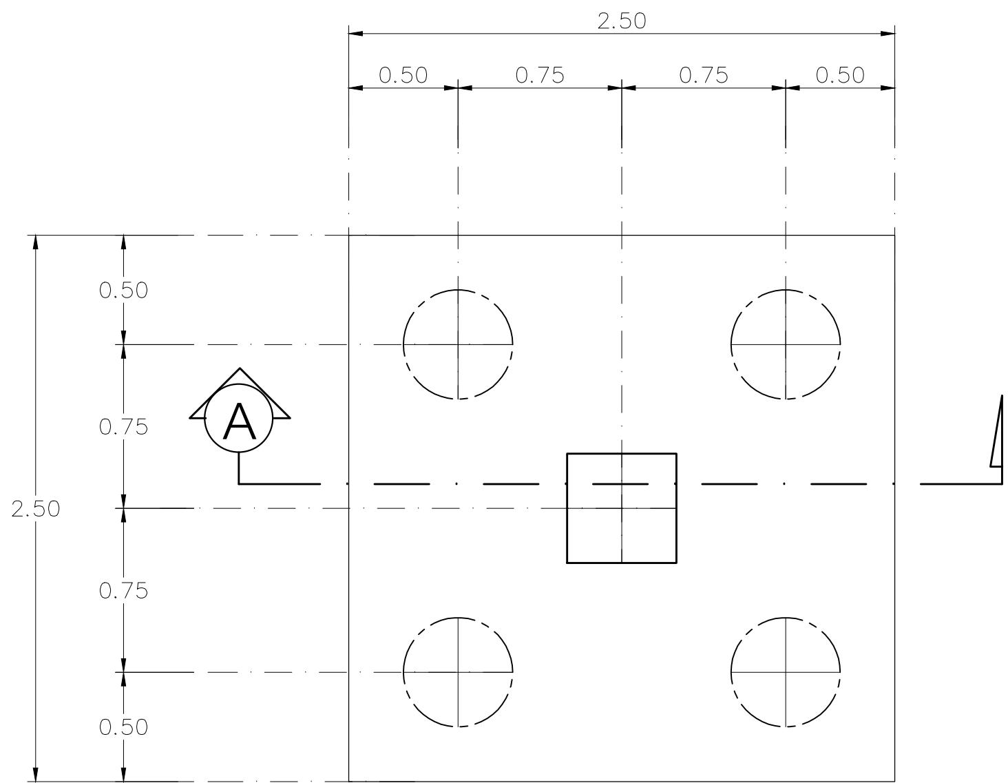
ขยายแปลนฐานราก F4 มาตราส่วน 1:25
