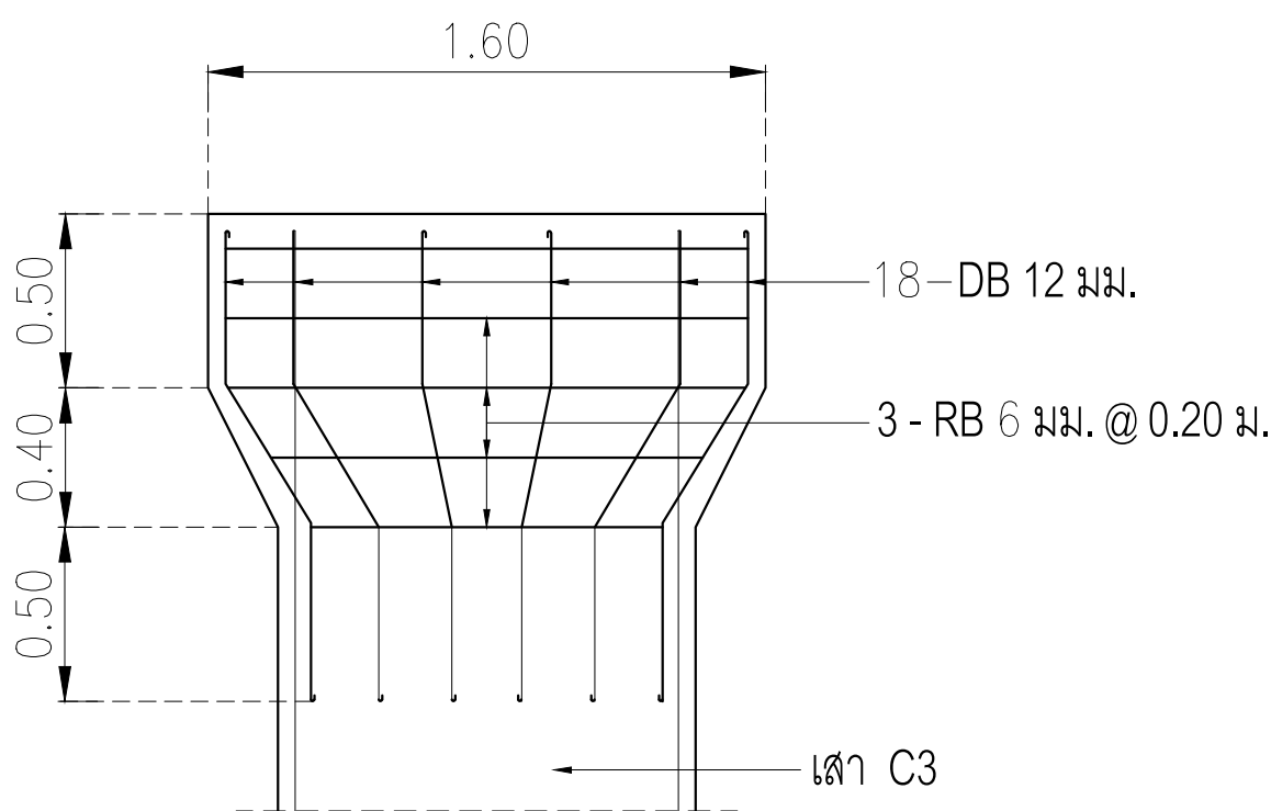
แบบขยายหัวเสารับหลังคา C3
