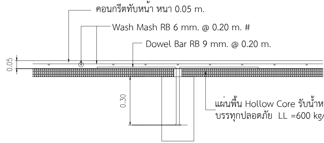
ขยายพื้น HC1
