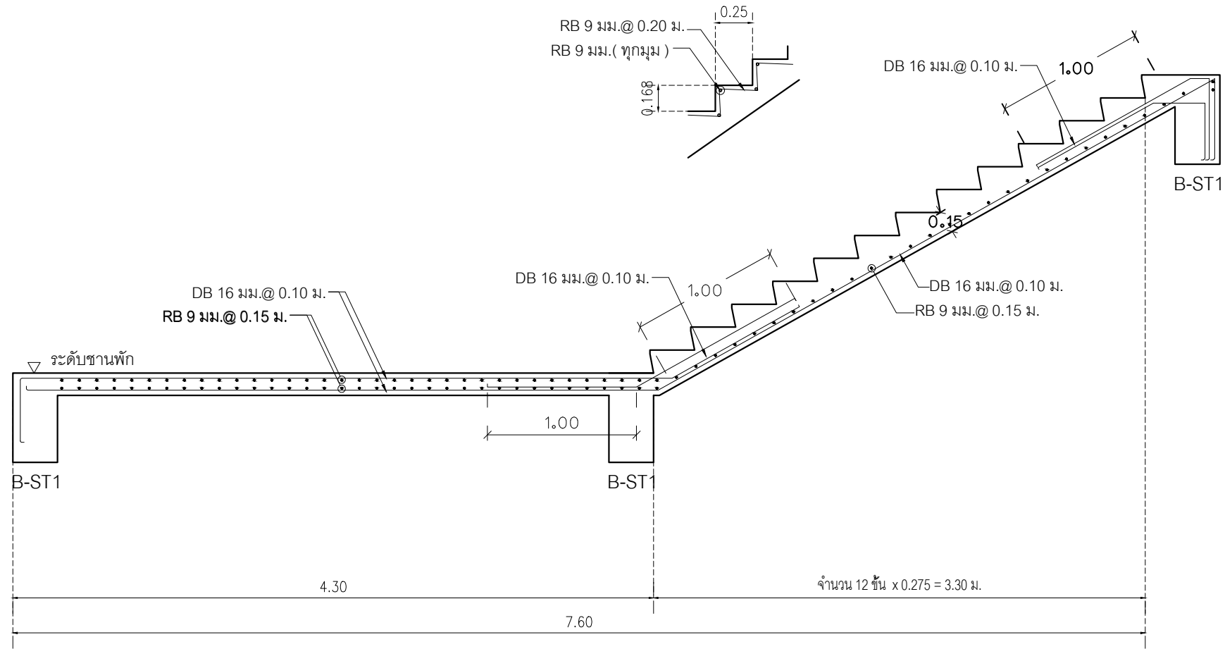
ST-1 ( ขานพัก - พื้น ) (บันไดหลัก)
