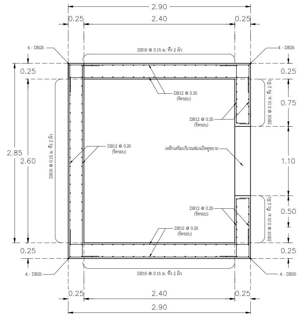
(ชั้นล่าง - ห้องเครื่อง)
