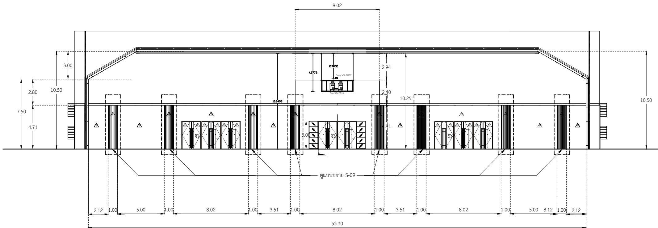
รูปด้าน D มาตราส่วน 1 : 200
