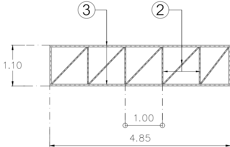
แบบขยาย T-13
