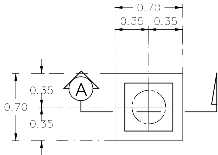
ขยายแปลนฐานราก F1A มาตราส่วน 1:25
