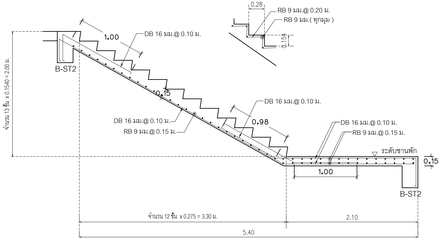
ST-2 ( ขานพัก - พื้น ) (บันไดหนีไฟ)
