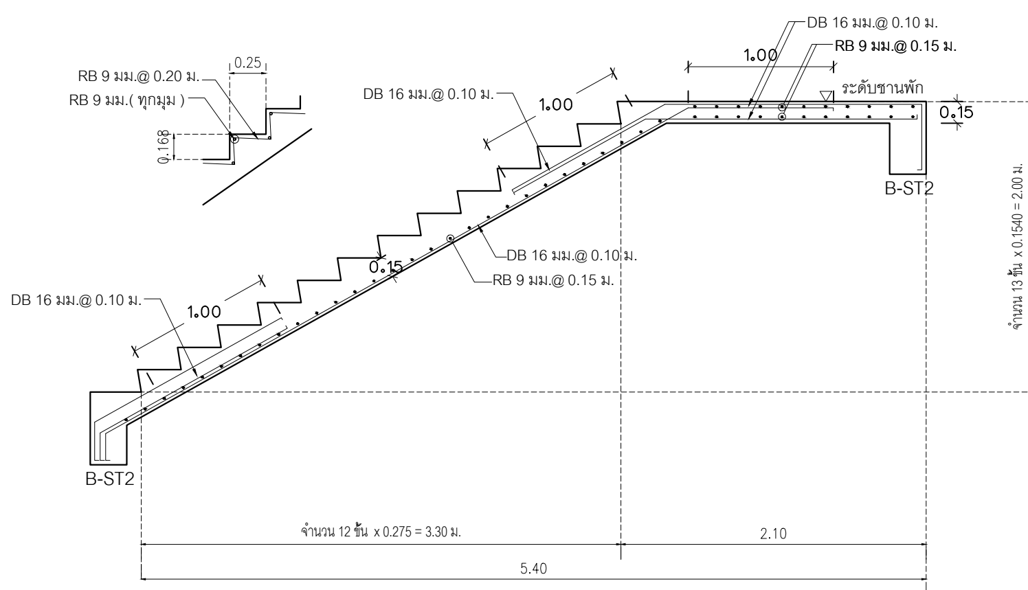
ST-2 ( พื้น - ขานพัก ) (บันไดหนีไฟ)
