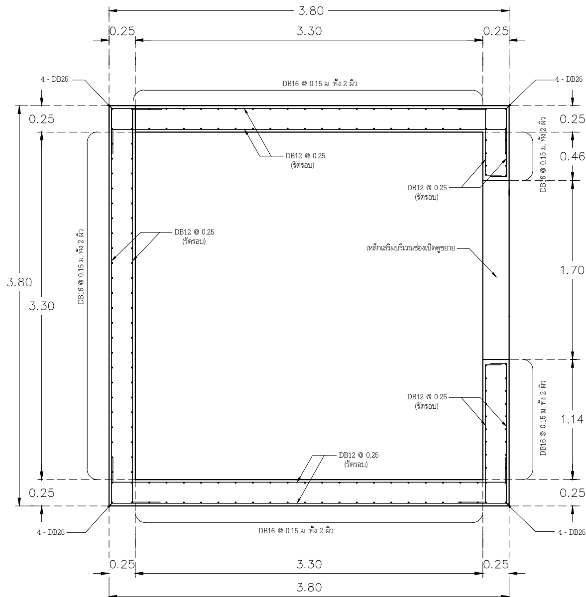
( ชั้นล่าง - ห้องเครื่อง )
