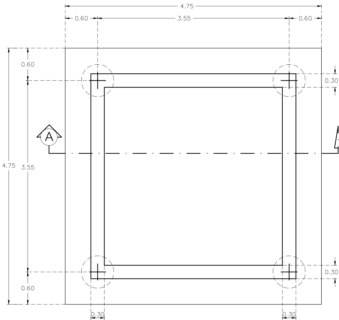
แปลน(ฐานราก )
