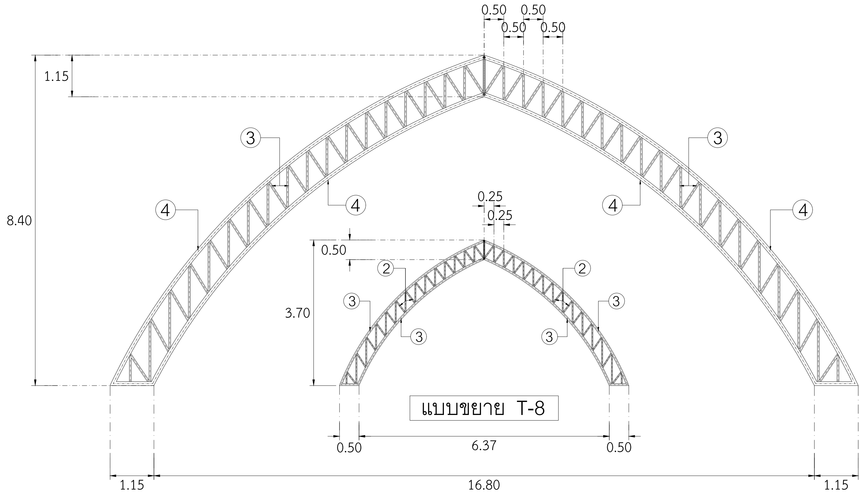
แบบขยาย T-7
