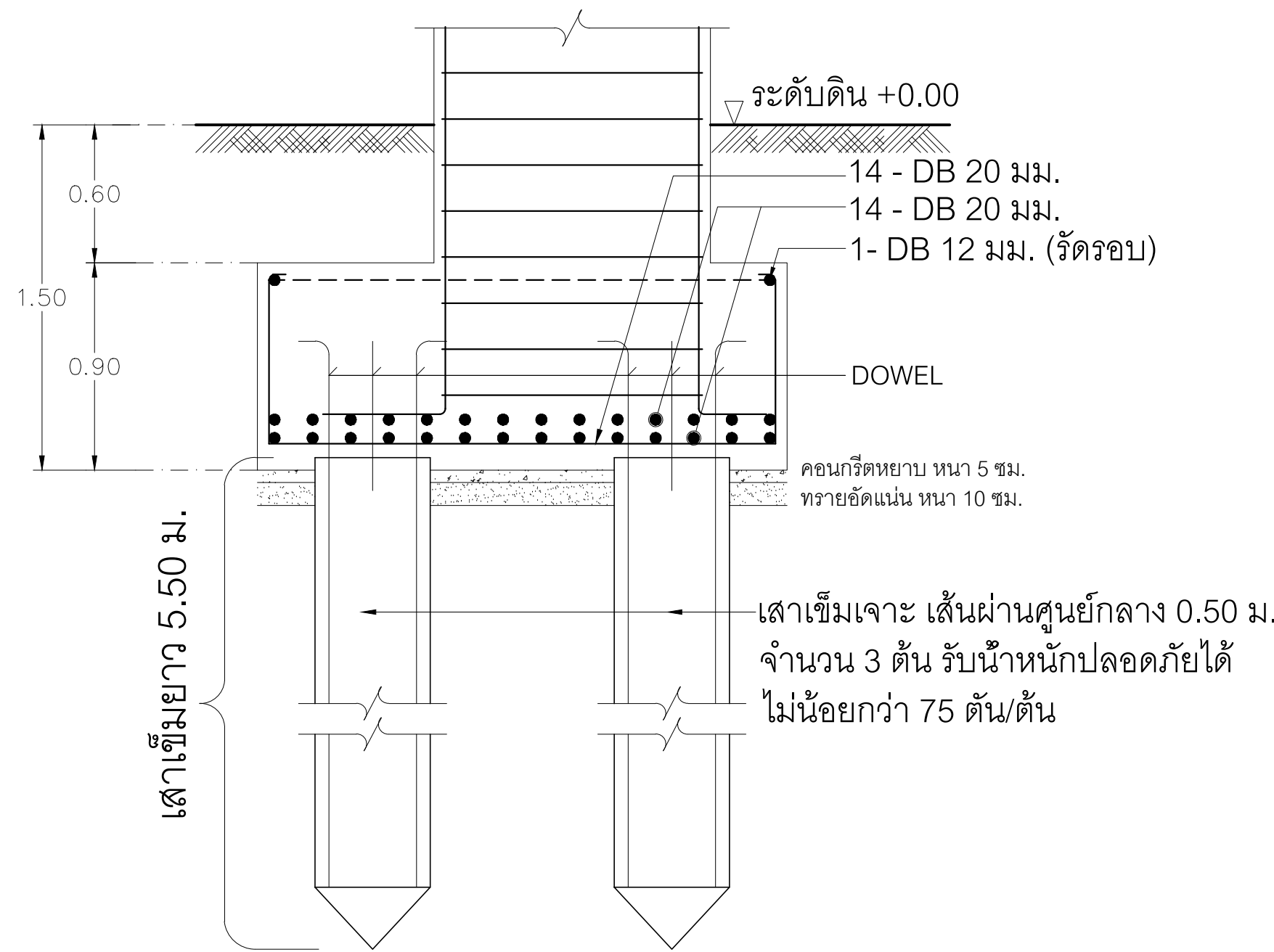
ขยายรูปตัด A มาตราส่วน 1:25
