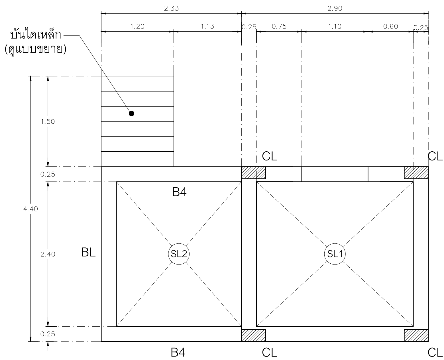
แปลนคานห้องเครื่องลิฟท์ มาตราส่วน 1 : 25
