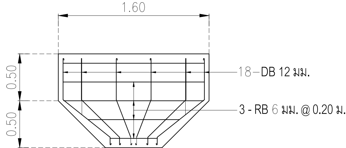
แบบขยายหัวคานรับโครงหลังคา T-1
