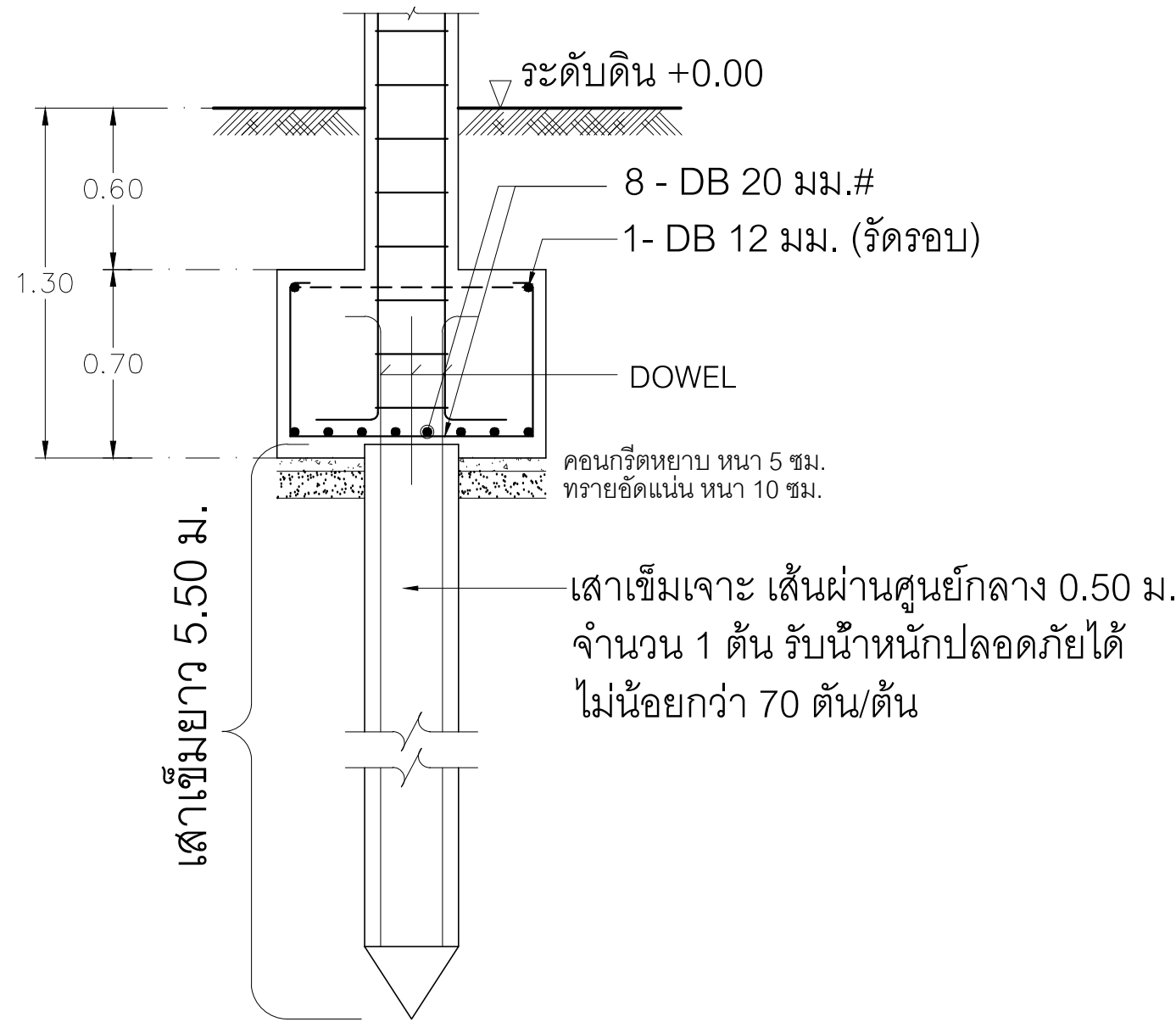
ขยายรูปตัด A มาตราส่วน 1:25
